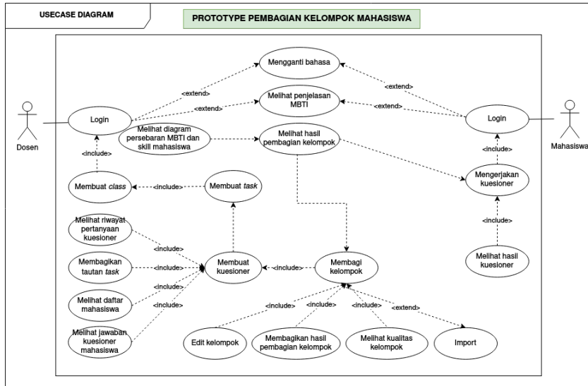
Gambar 3.2 Use Case Diagram Sistem Pembagian Kelompok
