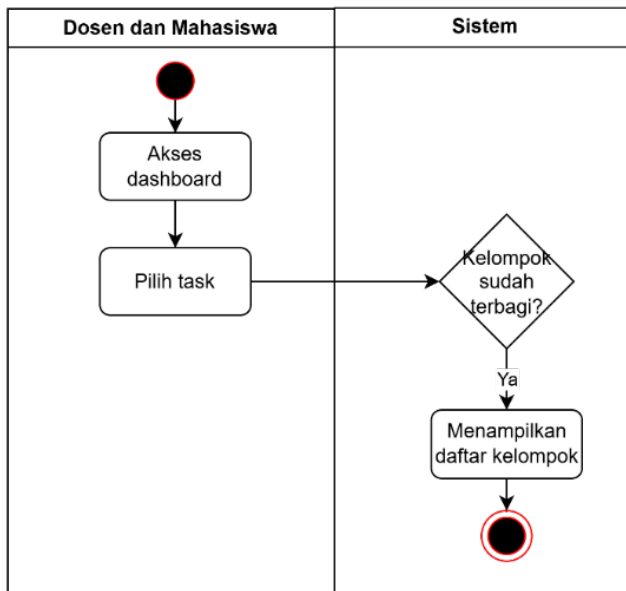
Gambar 3.6 Activity Diagram Melihat Hasil Pembagian Kelompok
