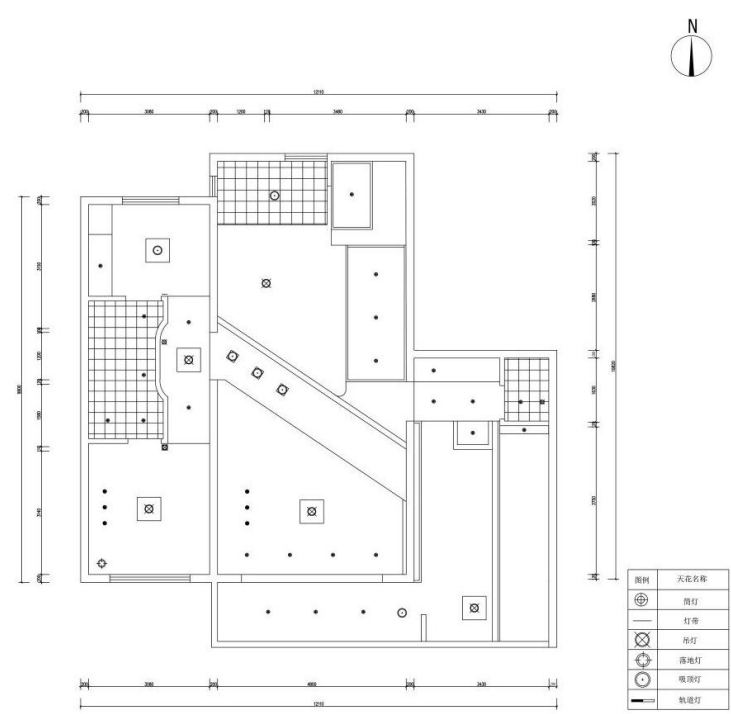
天花布置图
