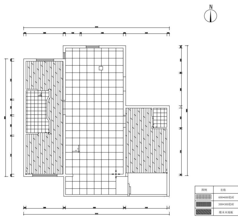
地面铺装图
