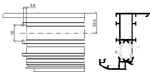
Asportazione dentini per passaggio asta
