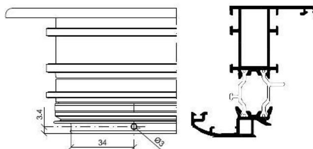
Squadretta a cianfrinare tubolare esterno anta
