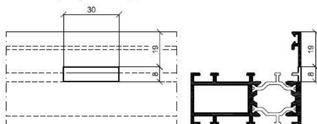
Scarico acqua (TP 8014)
