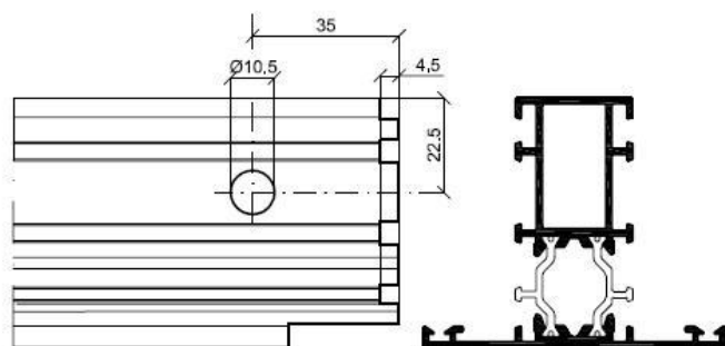
Cavallotto estruso (SQ 8028)
