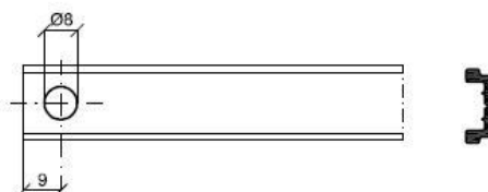
Foratura astina
