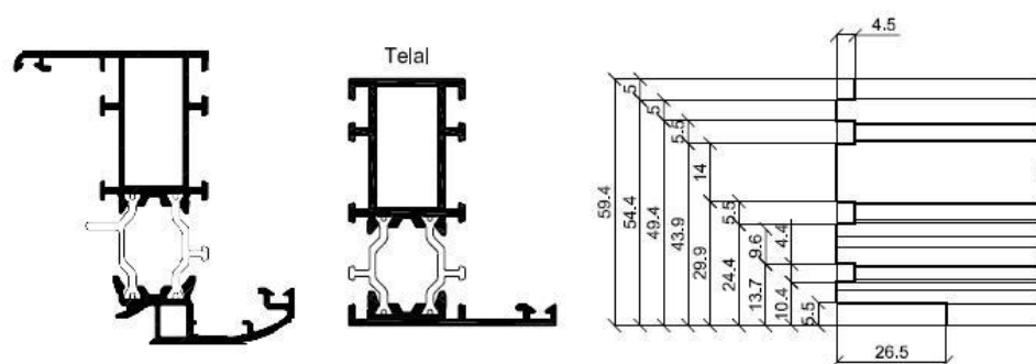
Fresatura fasce e zoccoli
