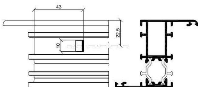
Squadretta multifunzione (cianfrinare)
