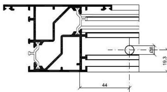
Asportazione dentini per passaggio asta
