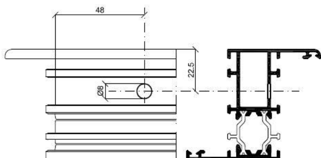
Squadretta multifunzione (spinare/avvitare)
