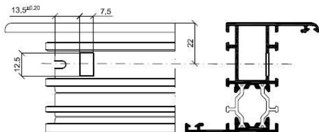
Squadretta in alluminio estruso
