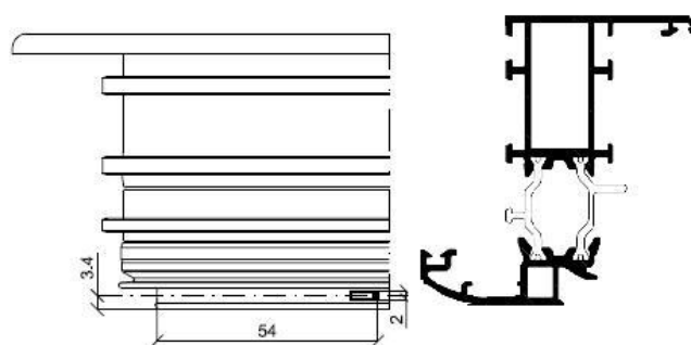
Squadretta con aggancio interno a vite
