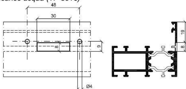
Scarico acqua (TP 8016)
