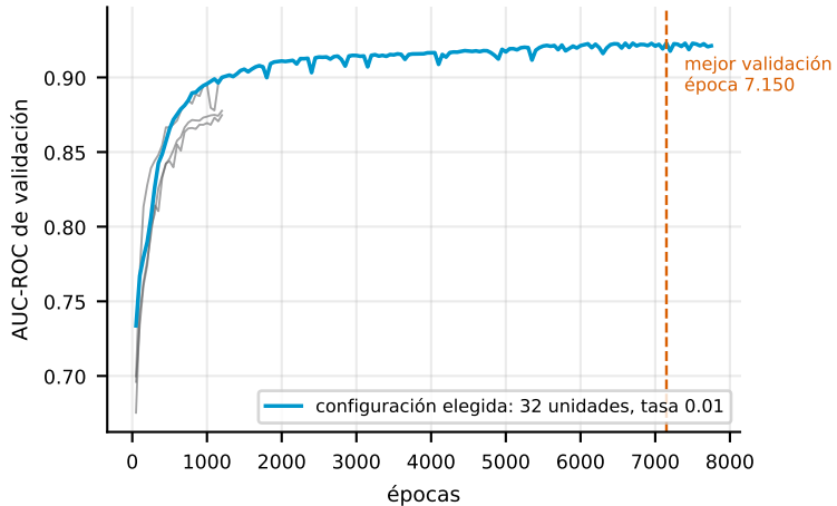
GCN de dos capas
