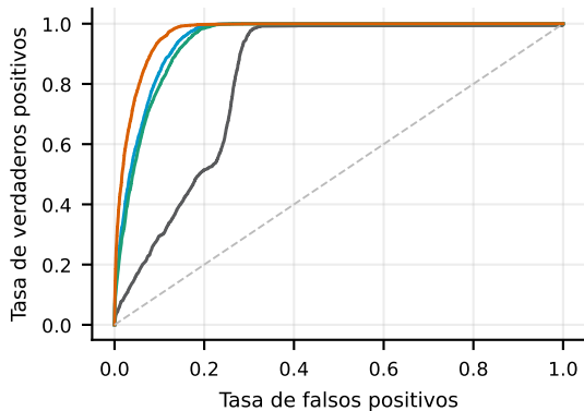
Curva ROC
