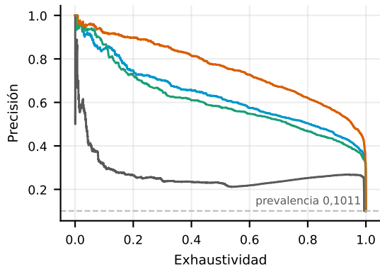
Curva precisión-exhaustividad
