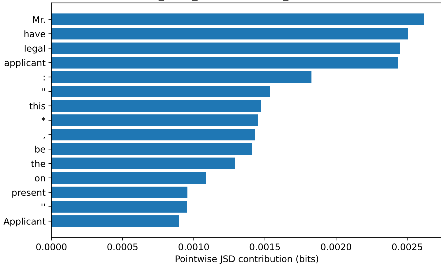
euro_court_cases: gemma2_9b vs human
