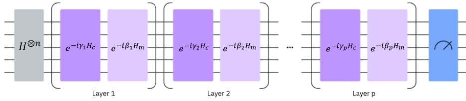
Estructura de Capas Alternadas en el Algoritmo QAOA
