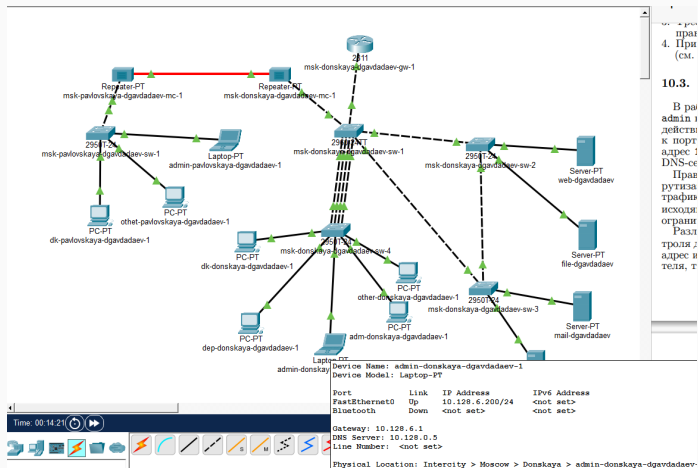
Рис. 1: Подключение и настройка ноутбука администратора
