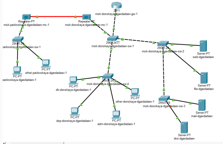
Рис. 1: Топология сети с DNS-сервером
