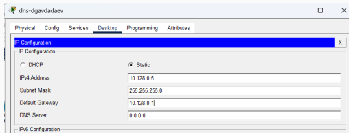
Рис. 2: Настройка IP DNS-сервера
