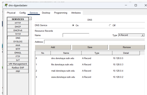
Рис. 3: Настройка службы DNS
