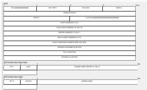
Рис. 12: DHCP ACK
