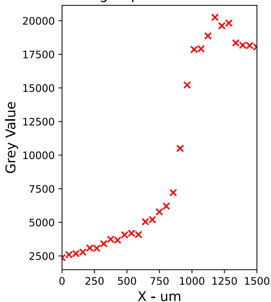
Edge Spread Function
