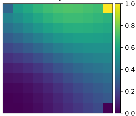
Unmixed Abundances
