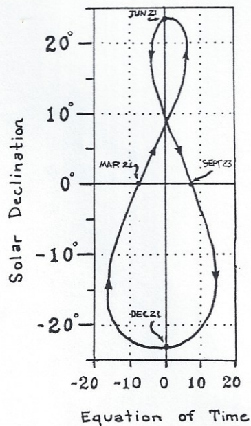
SOLAR ANALEMMA
