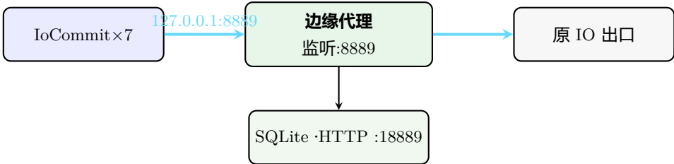
图 2: 边缘代理拦截 IoCommit 流量，透明转发 + 记录
