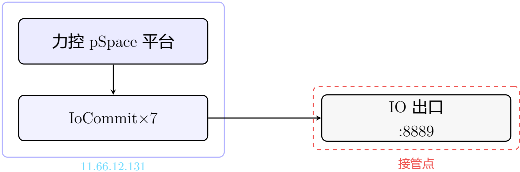
图 1: IoCommit×7 是 pSpace 对外的 IO 出口，在此插入代理
