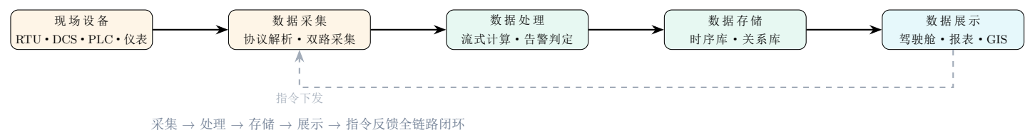
图 2: 数据流图—从现场设备到管理屏幕的抽象数据管道
