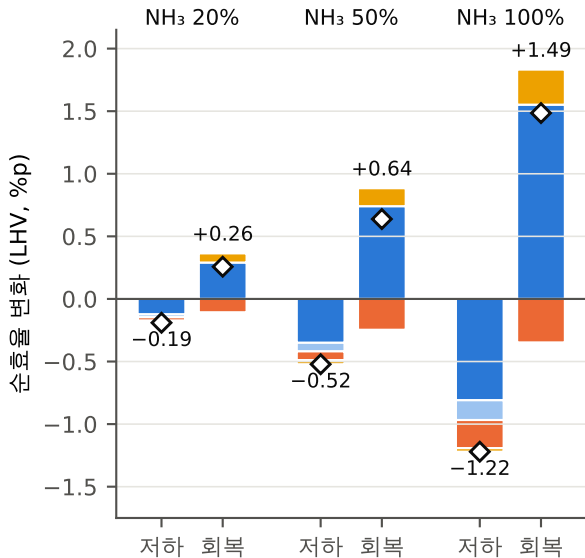
(b) LHV 기준
