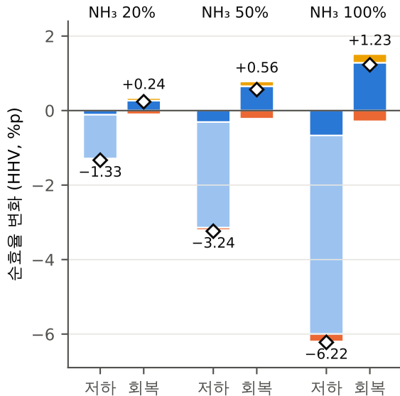
(c) HHV 기준
