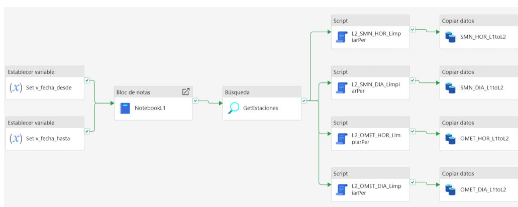
FIGURA 3.6. Pipeline de Fabric para la orquestación de datos meteorológicos observados.
