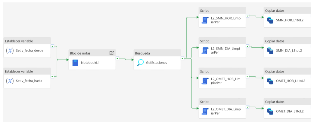
FIGURA 3.5. Pipeline de Fabric para la orquestación de datos meteorológicos.
