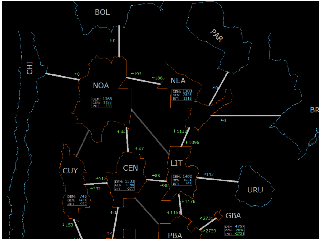
FIGURA 3.3. Generación e intercambios entre regiones. Imagen del SOTR de CAMMESA para un instante determinado.
