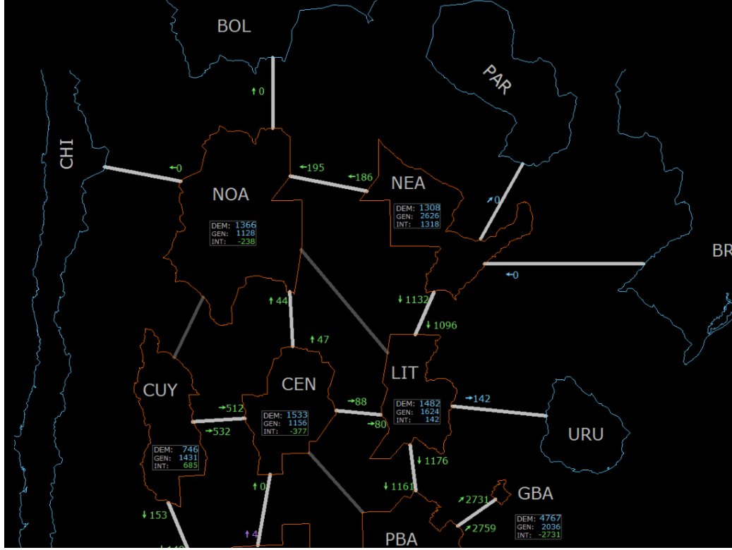
FIGURA 3.2. Generación e intercambios entre regiones. Imagen del SOTR de CAMMESA para un instante determinado.
