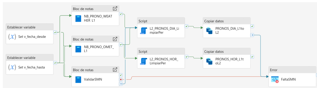
FIGURA 3.7. Pipeline de Fabric para la orquestación de pronósticos meteorológicos.
