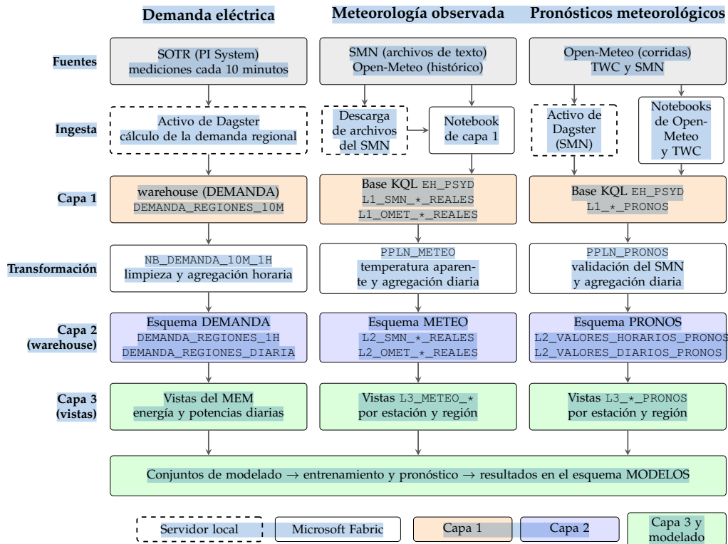
FIGURA 3.1. Diagrama general del pipeline de datos: flujos, etapas de procesamiento y capas de persistencia.
