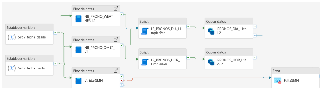
FIGURA 3.7. Pipeline de Fabric para la orquestación de pronósticos meteorológicos.
