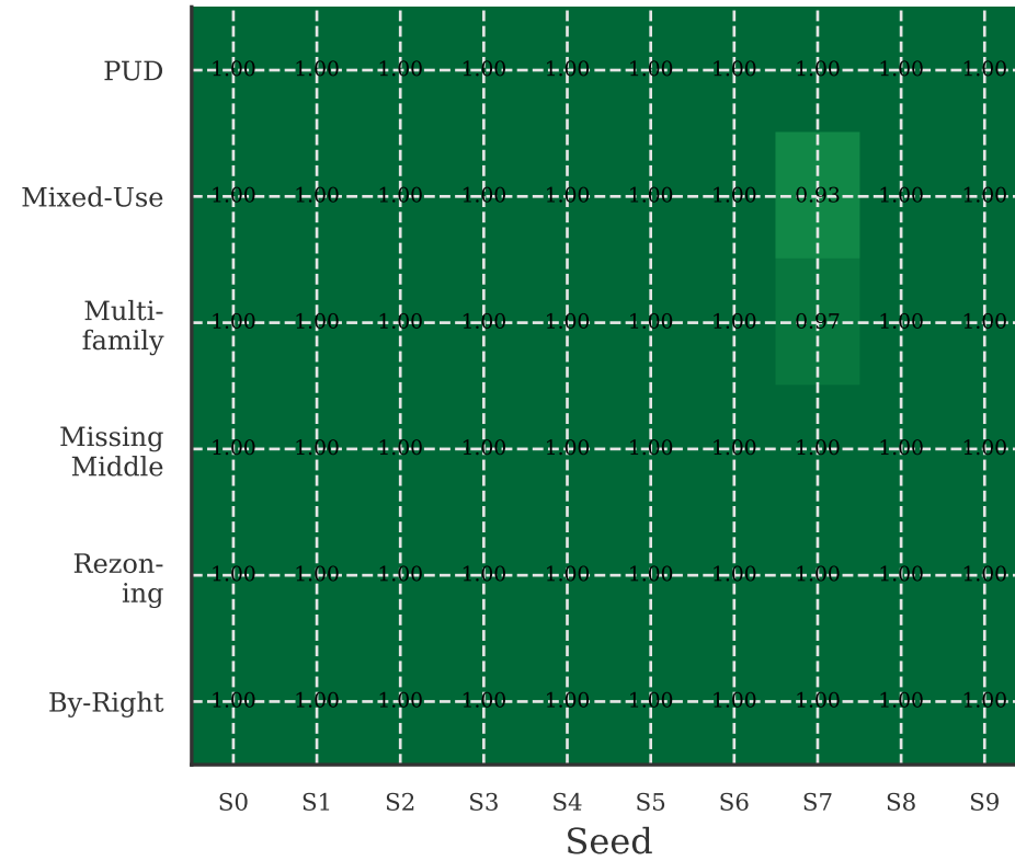
CatBoost
