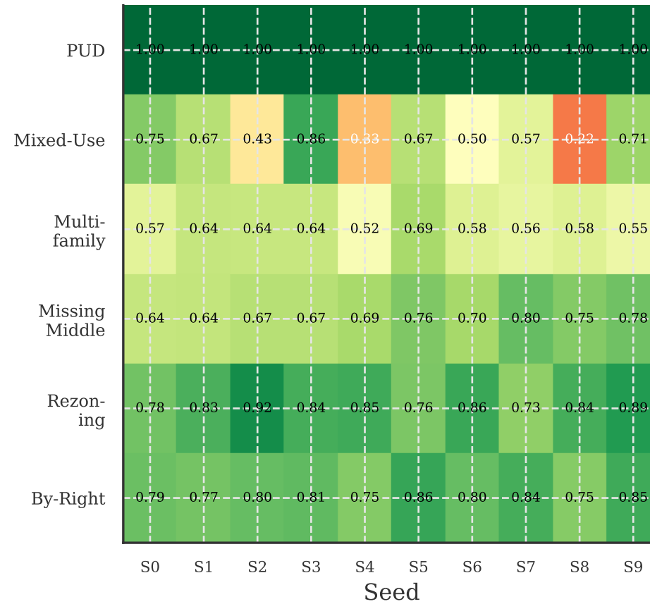
CatBoost
