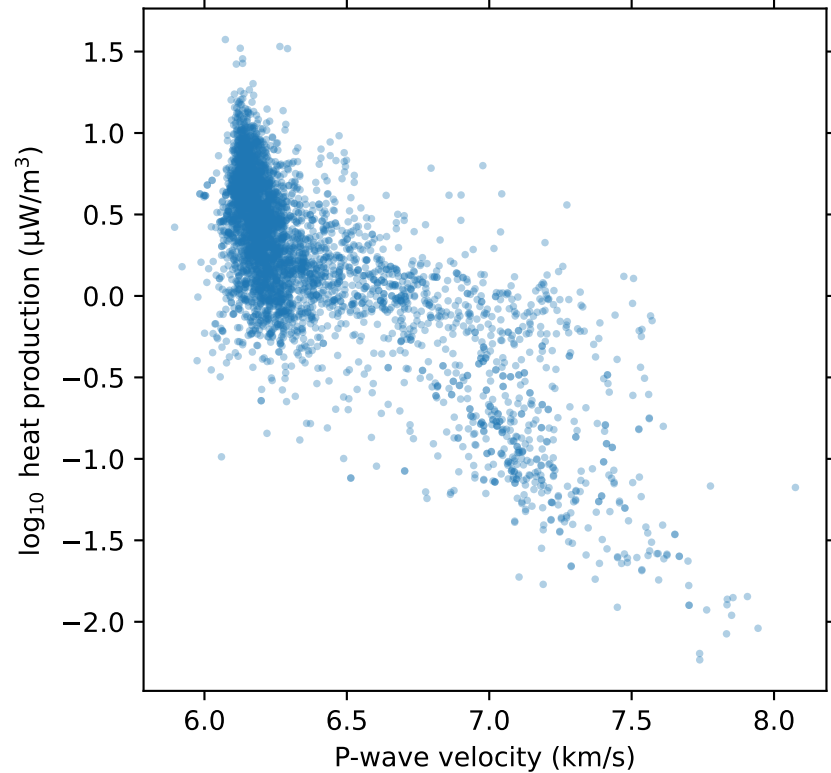
Yilgarn Craton
