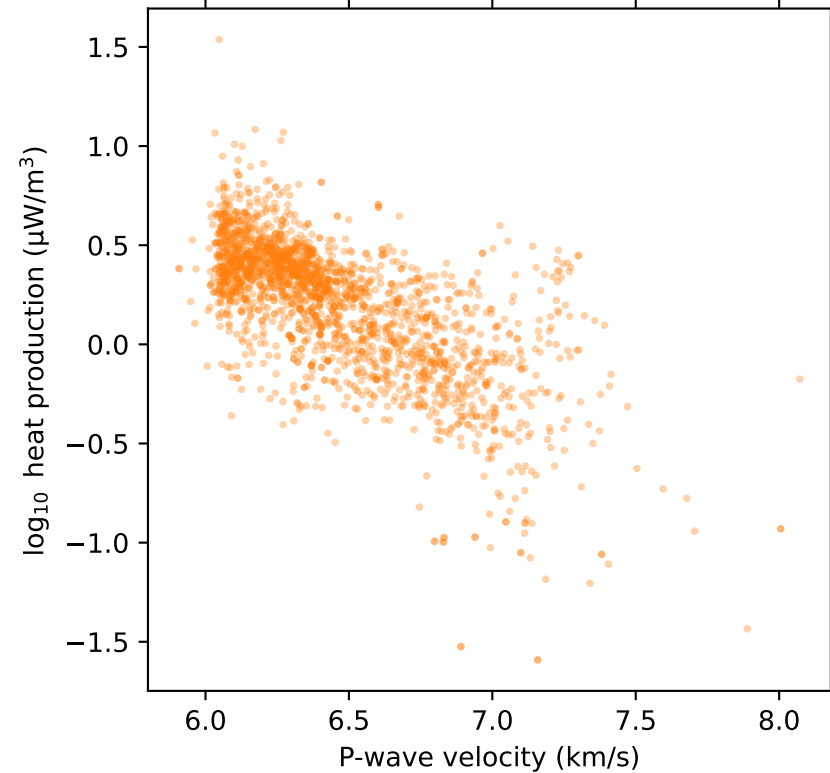
Macquarie Arc
