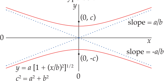
Hyperbola
