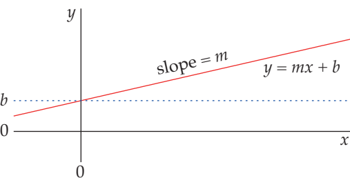
Linear
