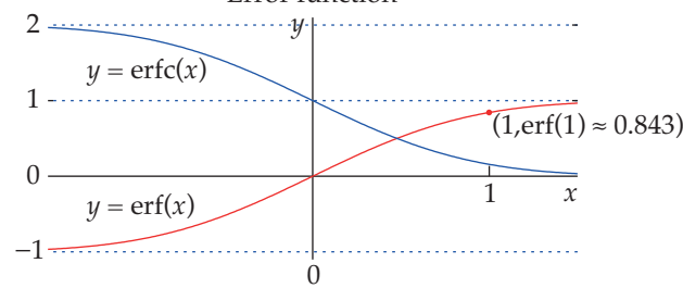
Error function
