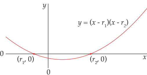
Parabola
