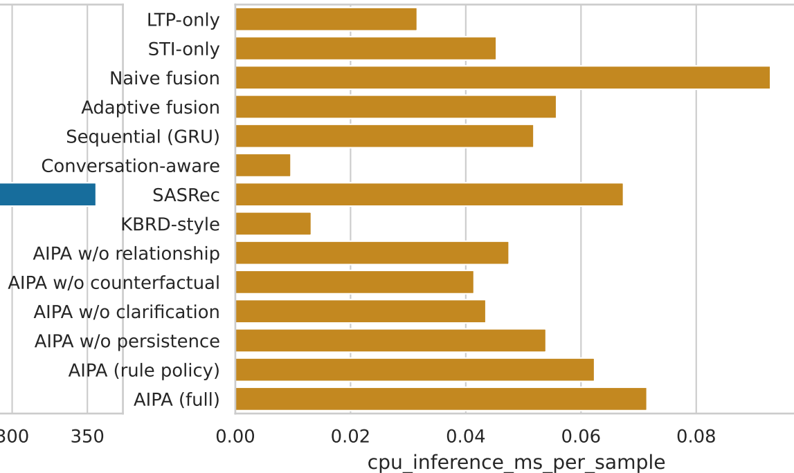
Inference time per test instance (ms)
