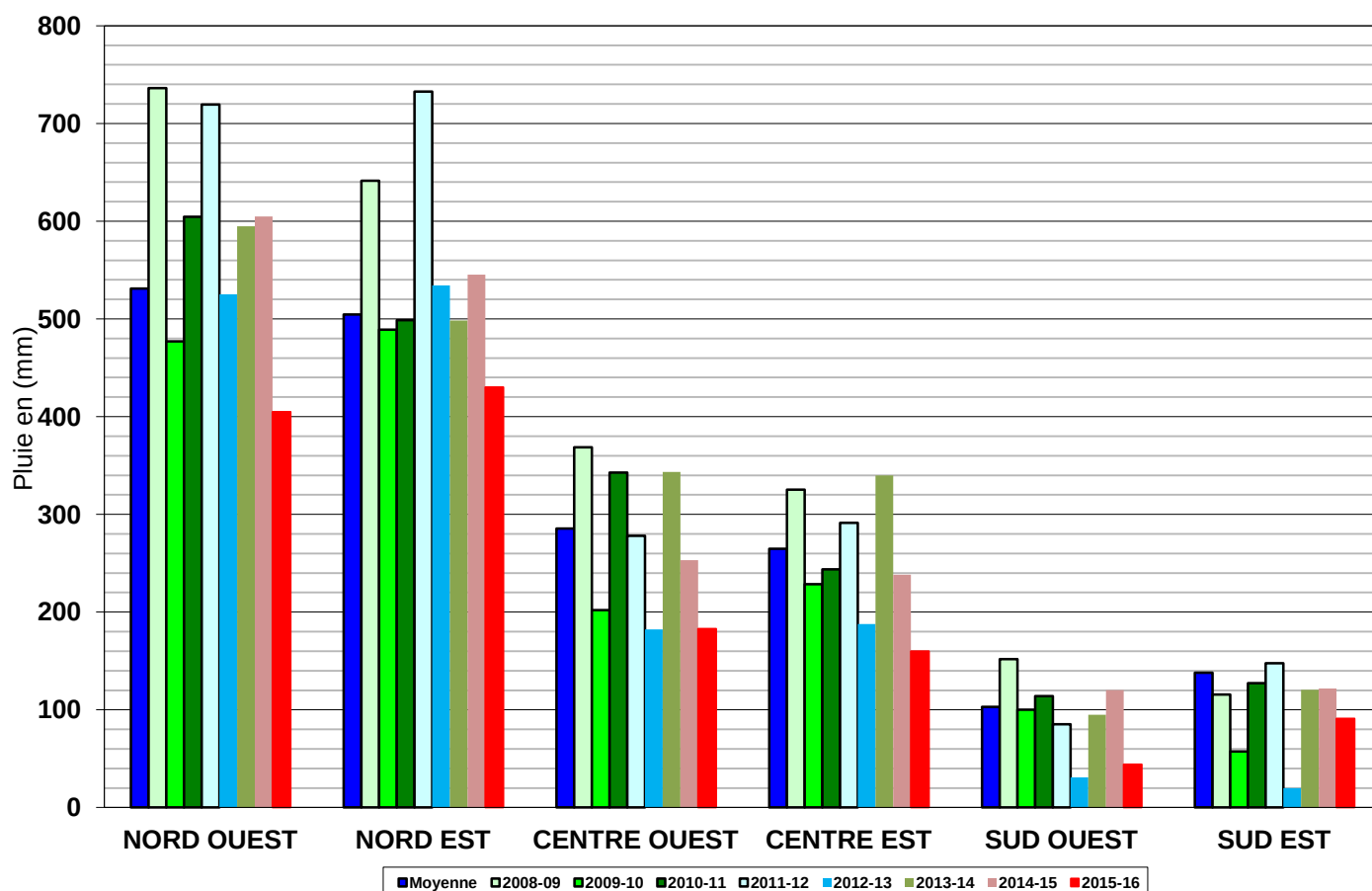
Figure 1 : Comparaison des pluviométries régionales des huit dernières années
