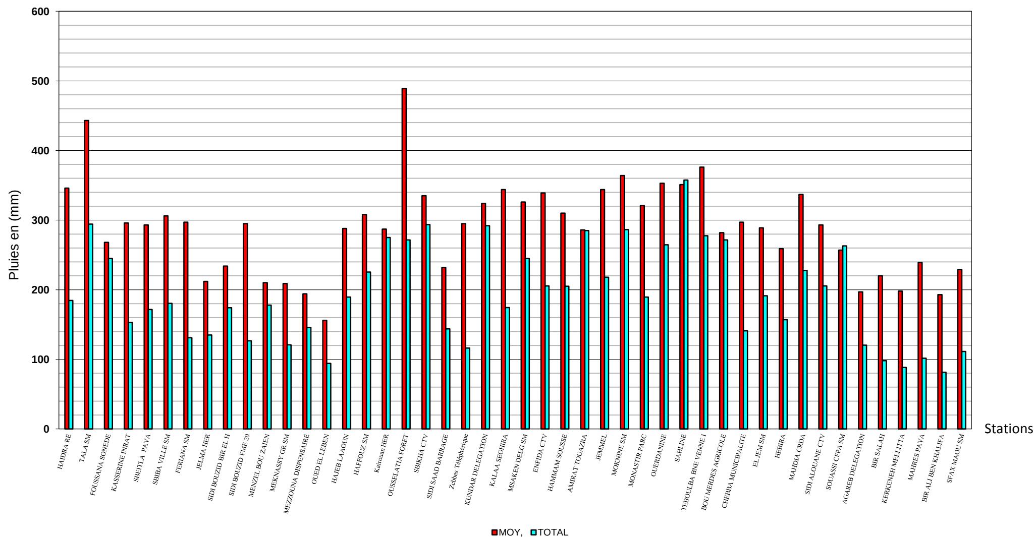
Figure 8: (Tunisie Centrale) : Pluviométrie annuelle 2015-2016 par station, comparée à la moyenne interannuelle
