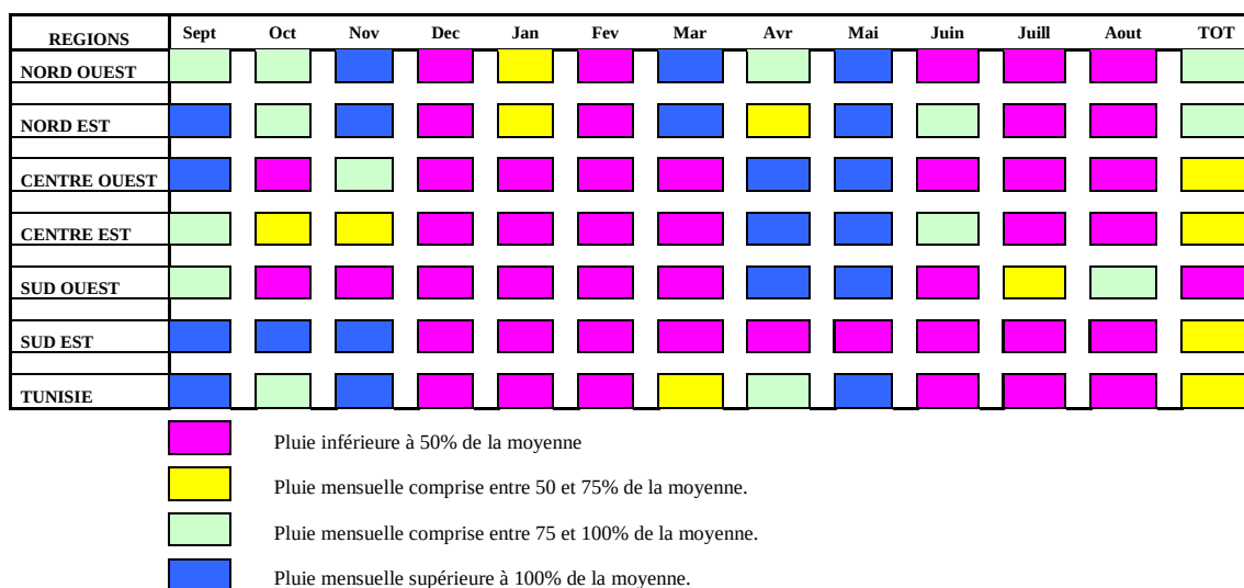
Figure 2 : Répartition des pluies mensuelles 2015-2016 par classe de pluviométrie
