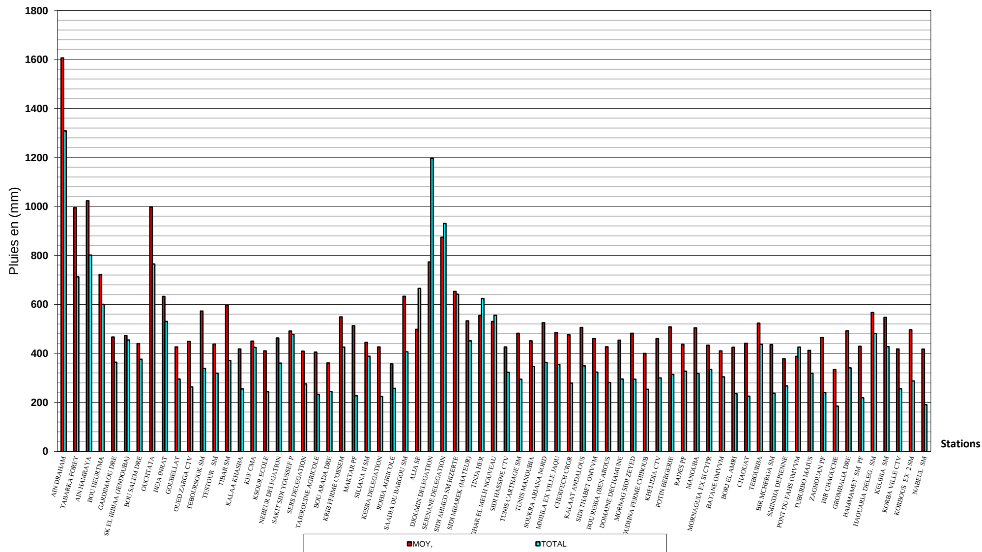
Figure 7: (Tunisie du Nord) : Pluviométrie annuelle 2015-2016 par station, comparée à la moyenne interannuelle
