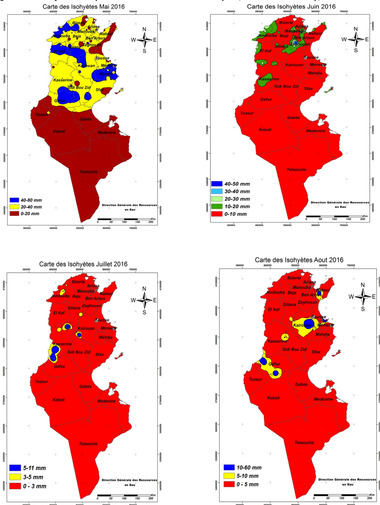
Figure 13: Isohyètes des pluies mensuelles des mois de (Mai, Juin Juil. et Août), année 2016
