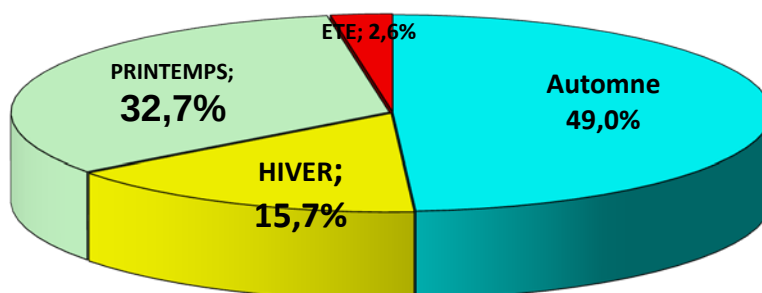
Figure 3 : Répartition des pluies saisonnières en % (Tunisie)
