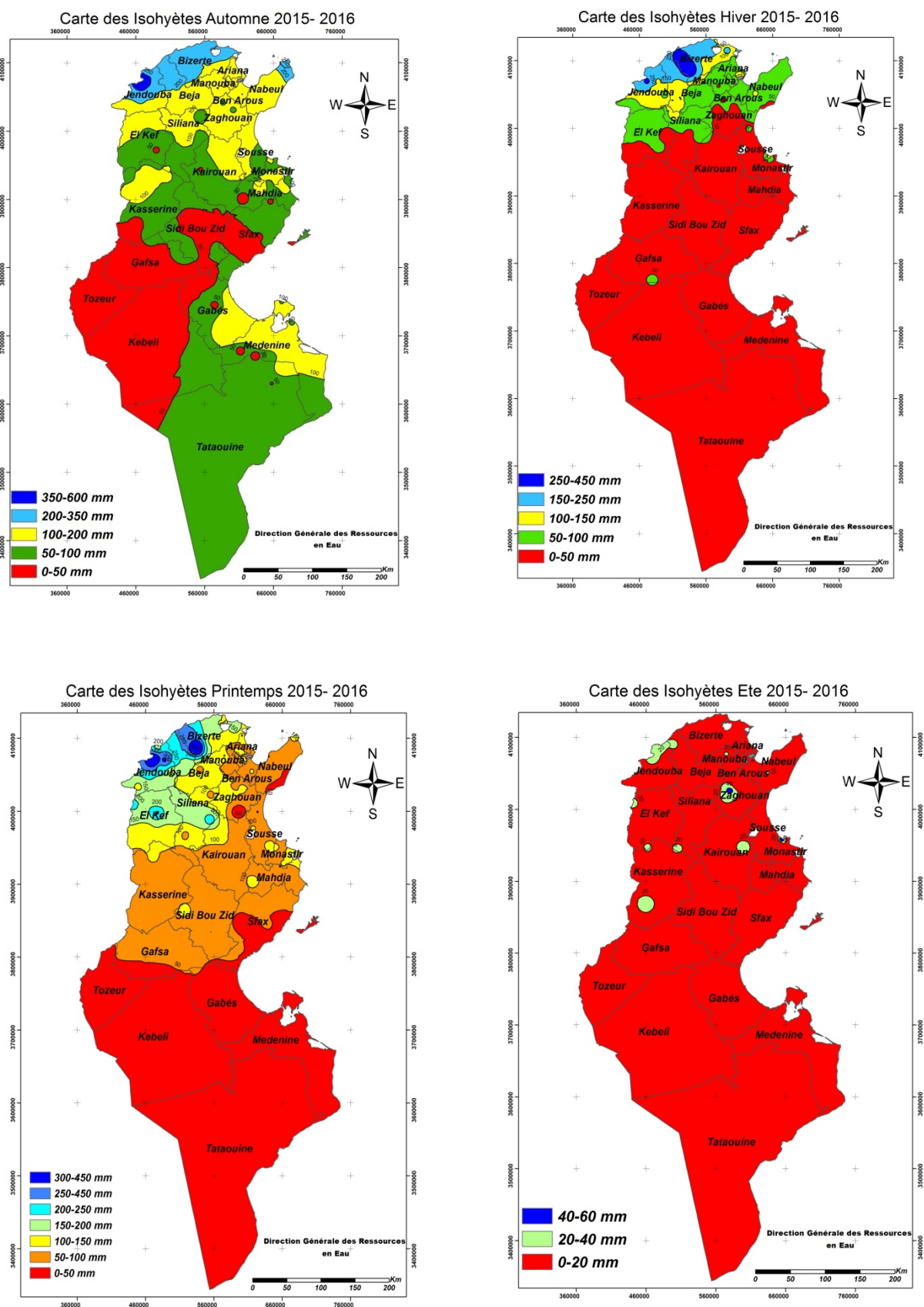
Figure 10: Isohyètes saisonnières de l'année 2015-2016
