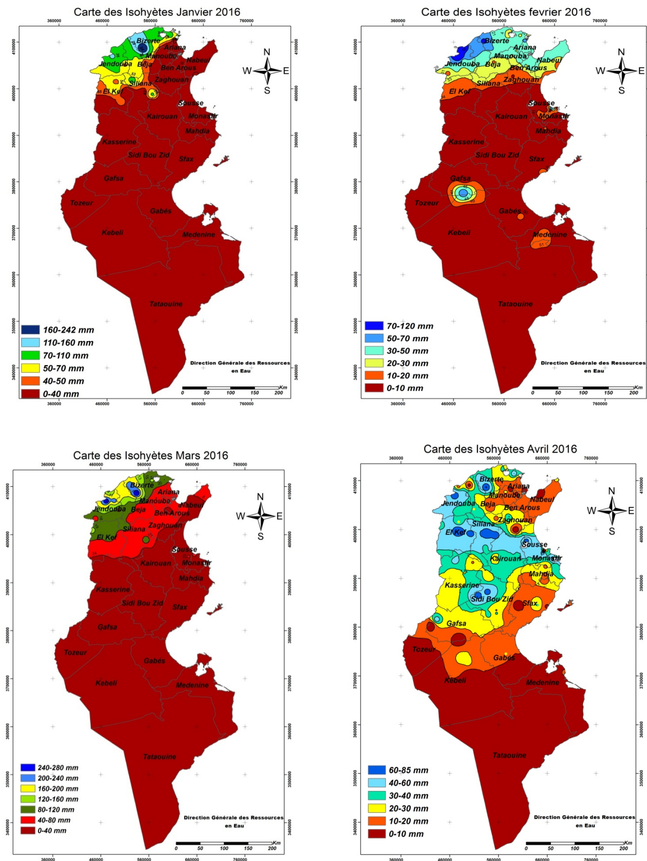
Figure 12 : Isohyètes des pluies mensuelles des mois de (Janv., Fév., Mars et Avril) ,année 2016
