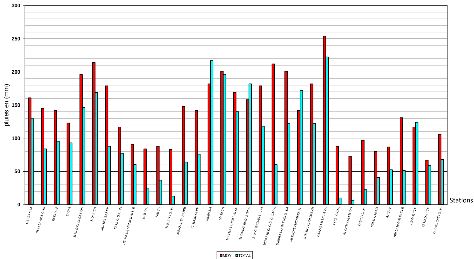
Figure 9: (Tunisie du Sud) : Pluviométrie annuelle 2015-2016 par station, comparée à la moyenne interannuelle
