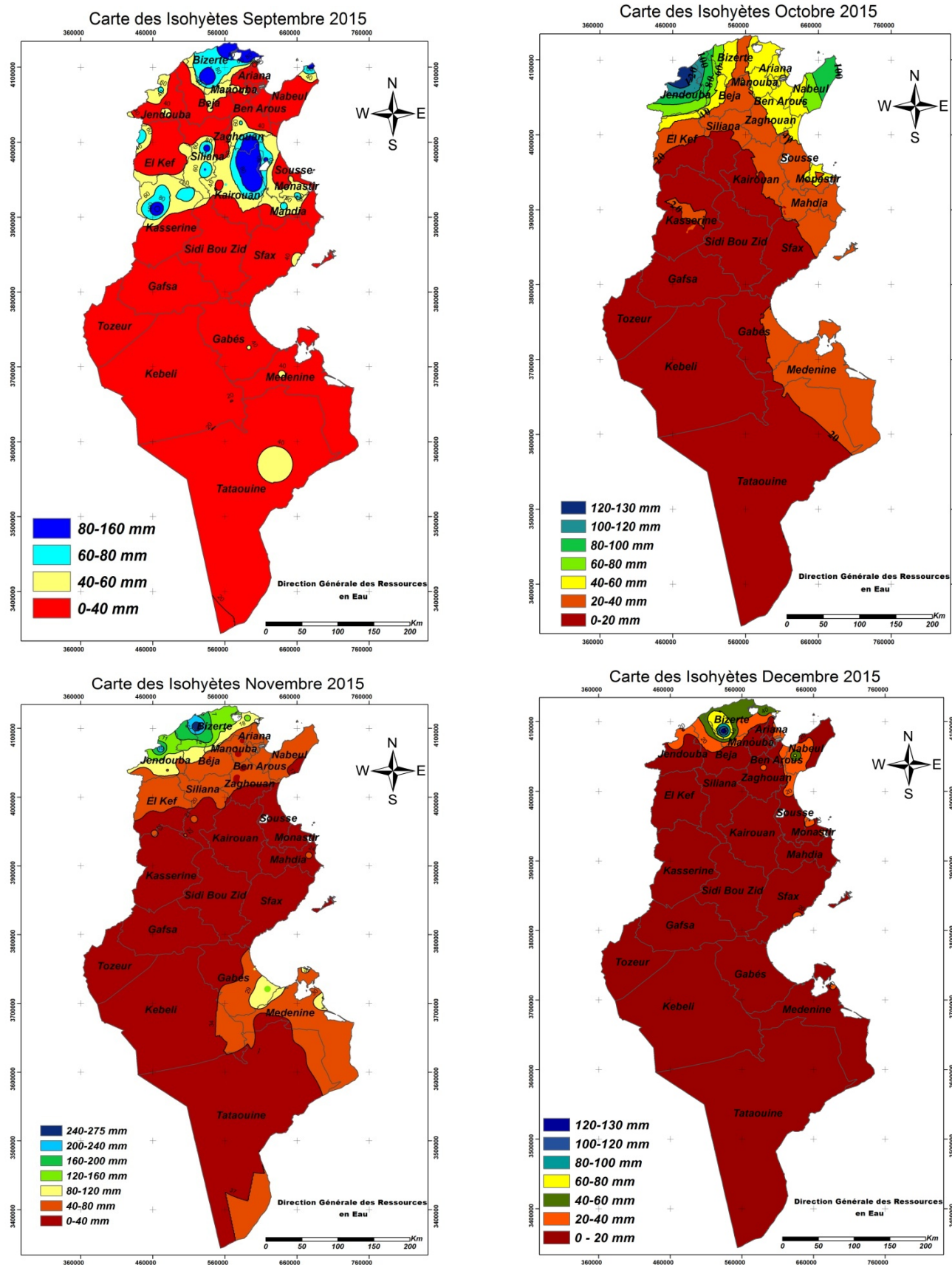
Figure 11: Isohyètes des pluies mensuelles des mois de (Sept., Oct., Nov. et Déc.) , année 2015
