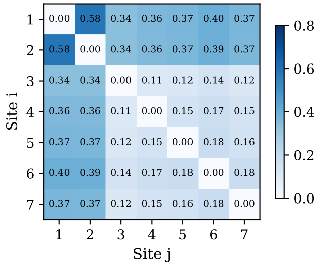
(b) QMI matrix (bits)
