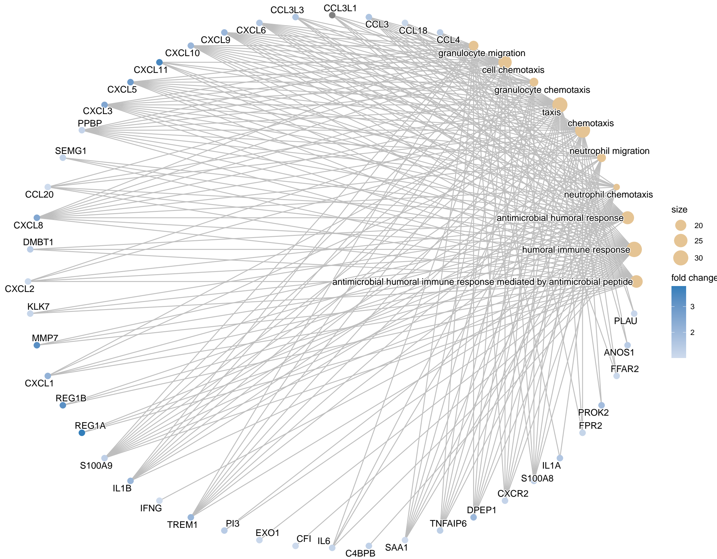
BP Cnetplot
