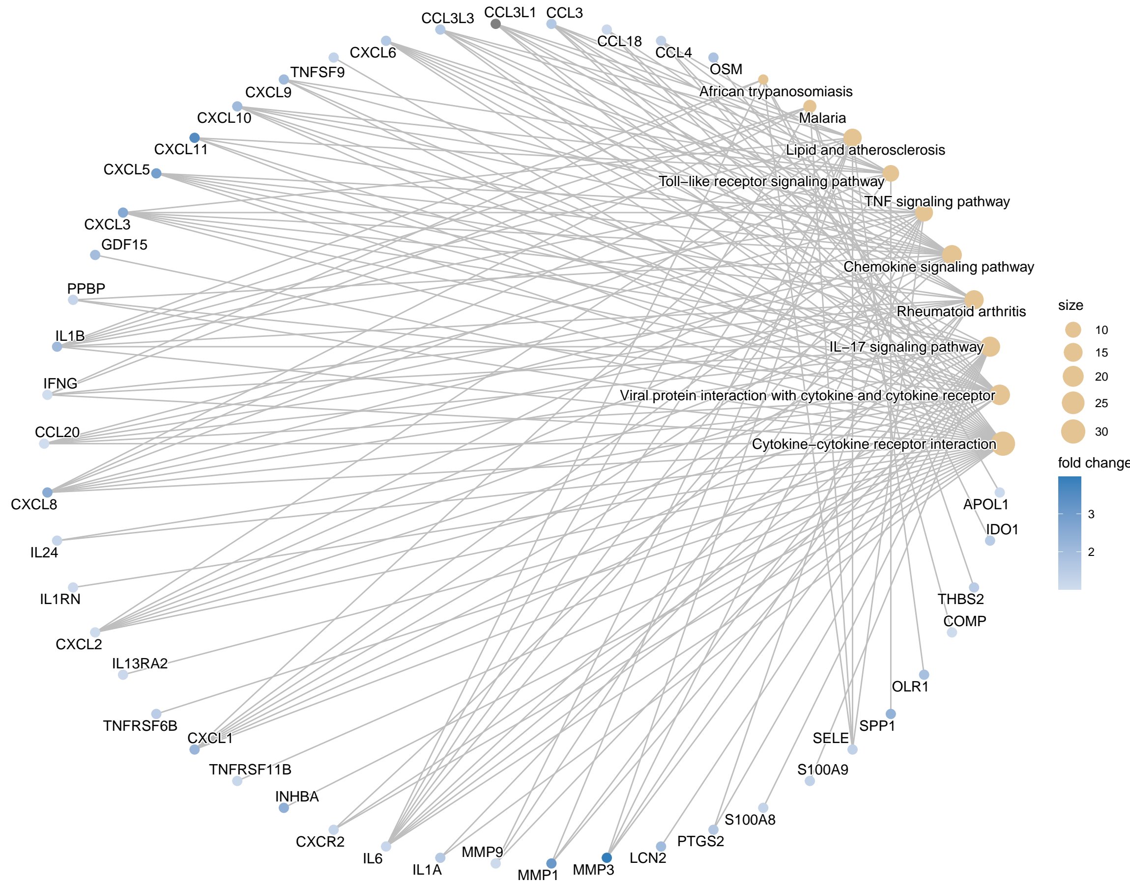
KEGG Cnetplot
