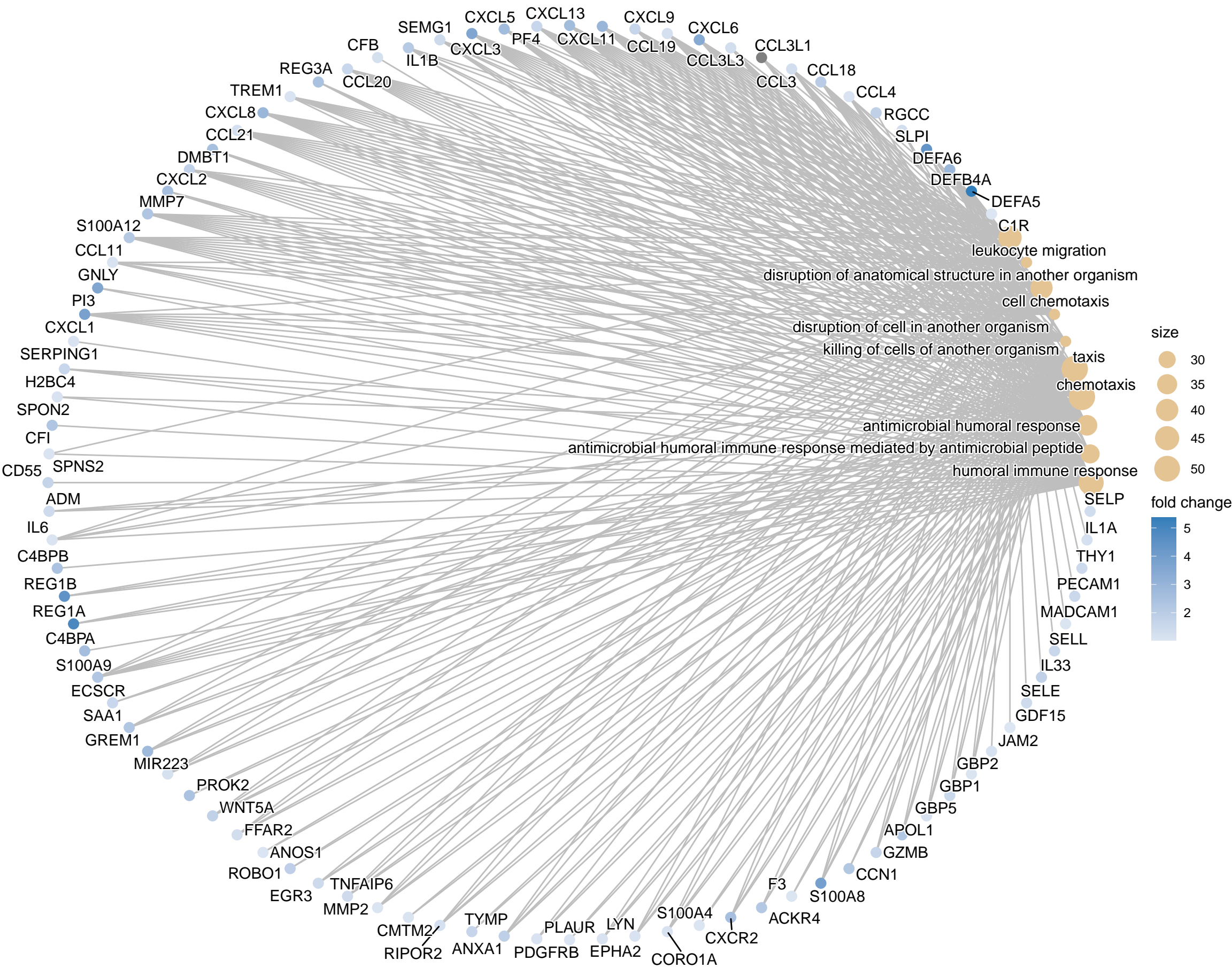
BP Cnetplot
