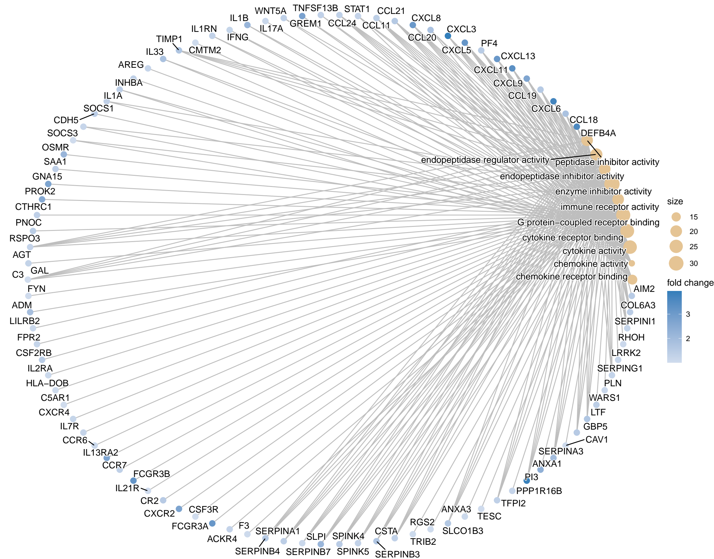
MF Cnetplot
