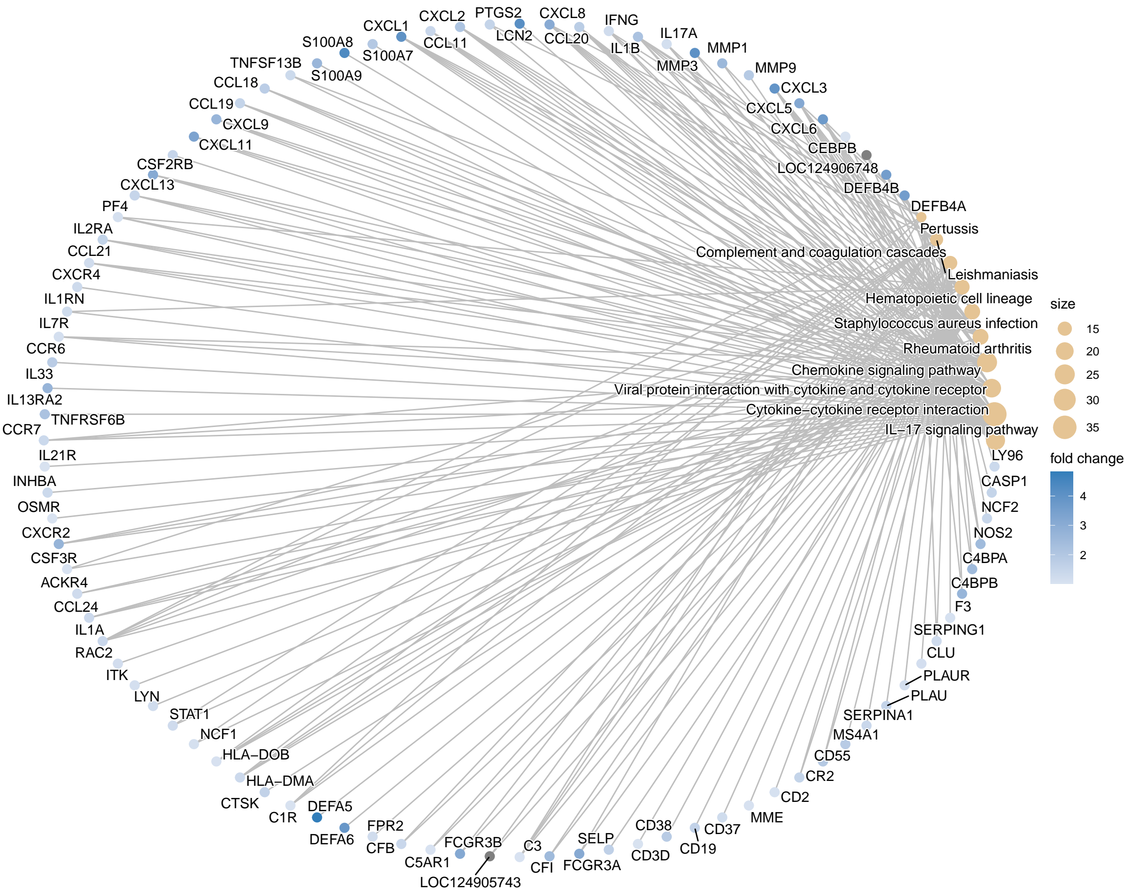
KEGG Cnetplot
