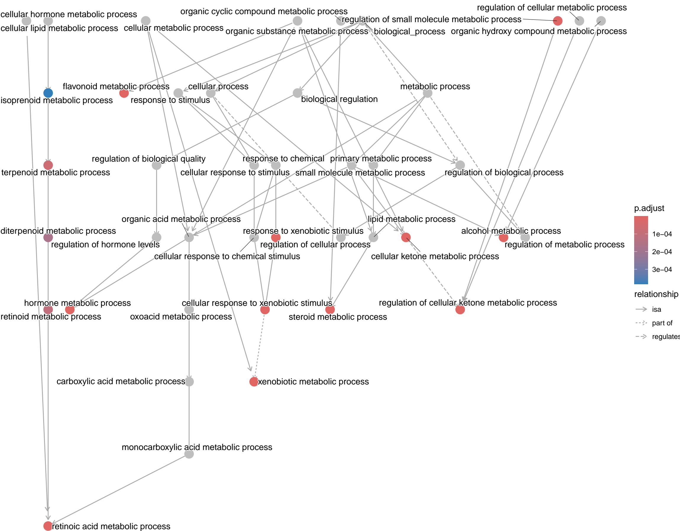
BP Goplot
