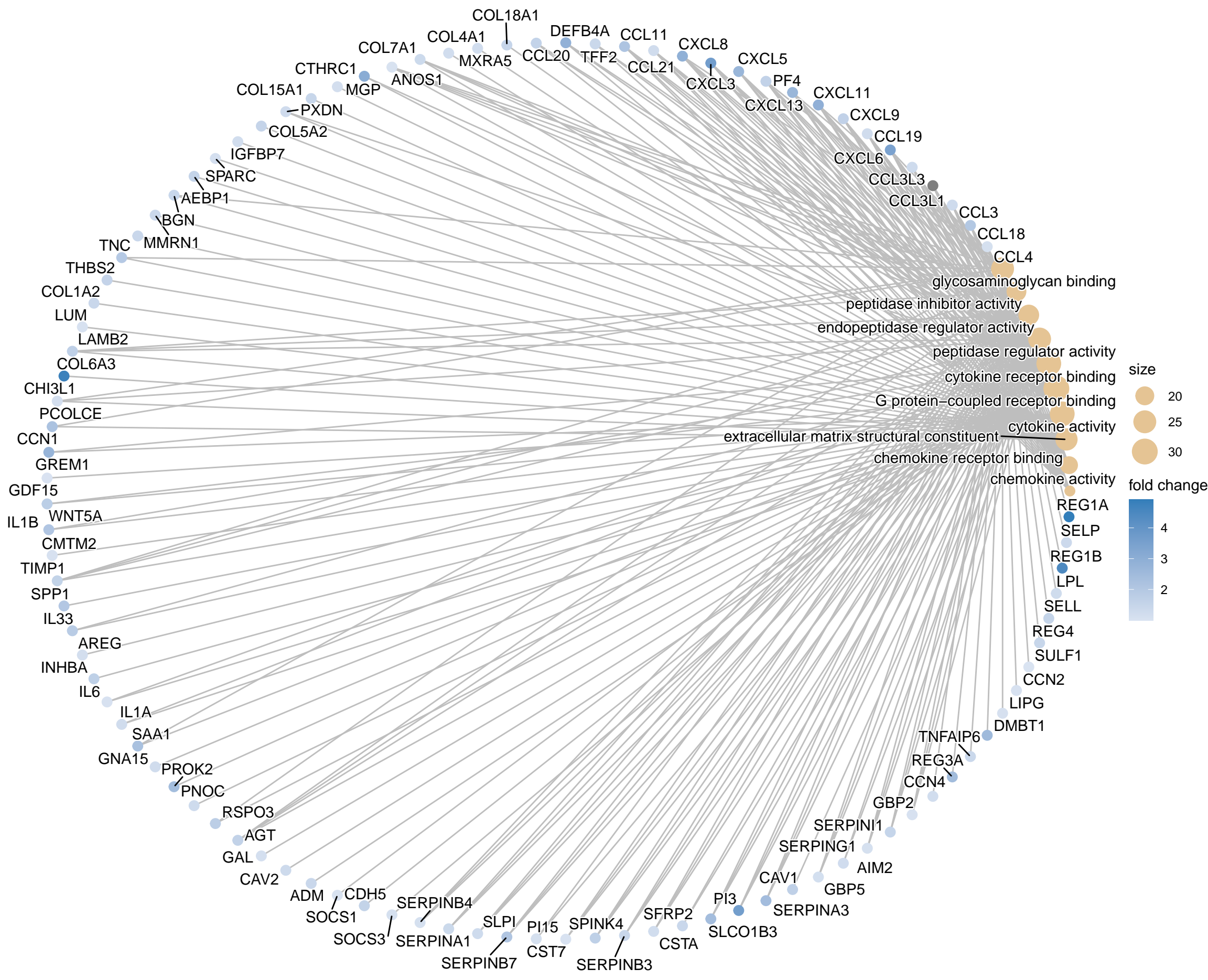
MF Cnetplot
