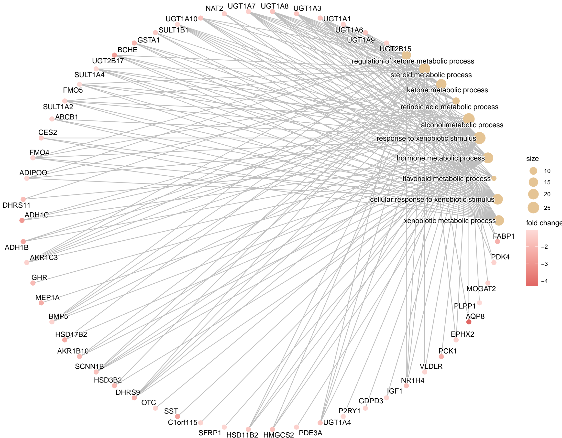
BP Cnetplot
