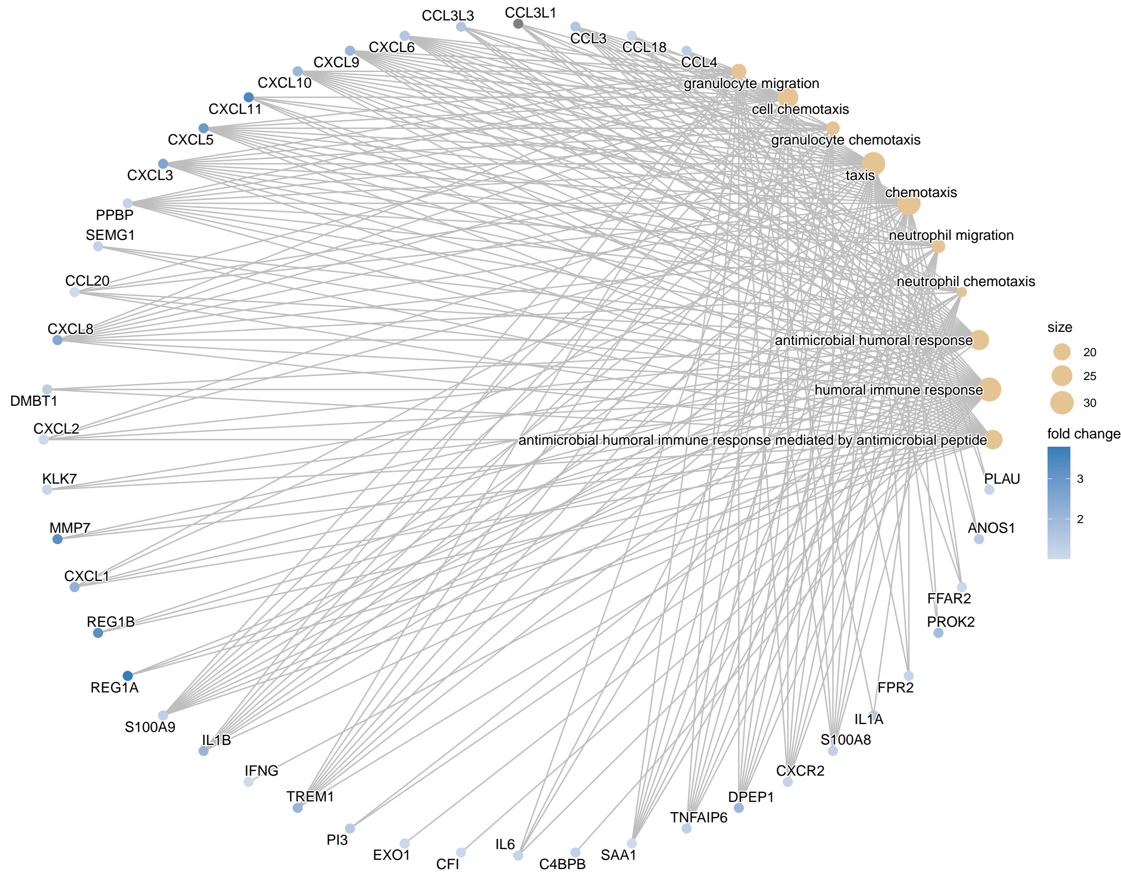
BP Cnetplot
