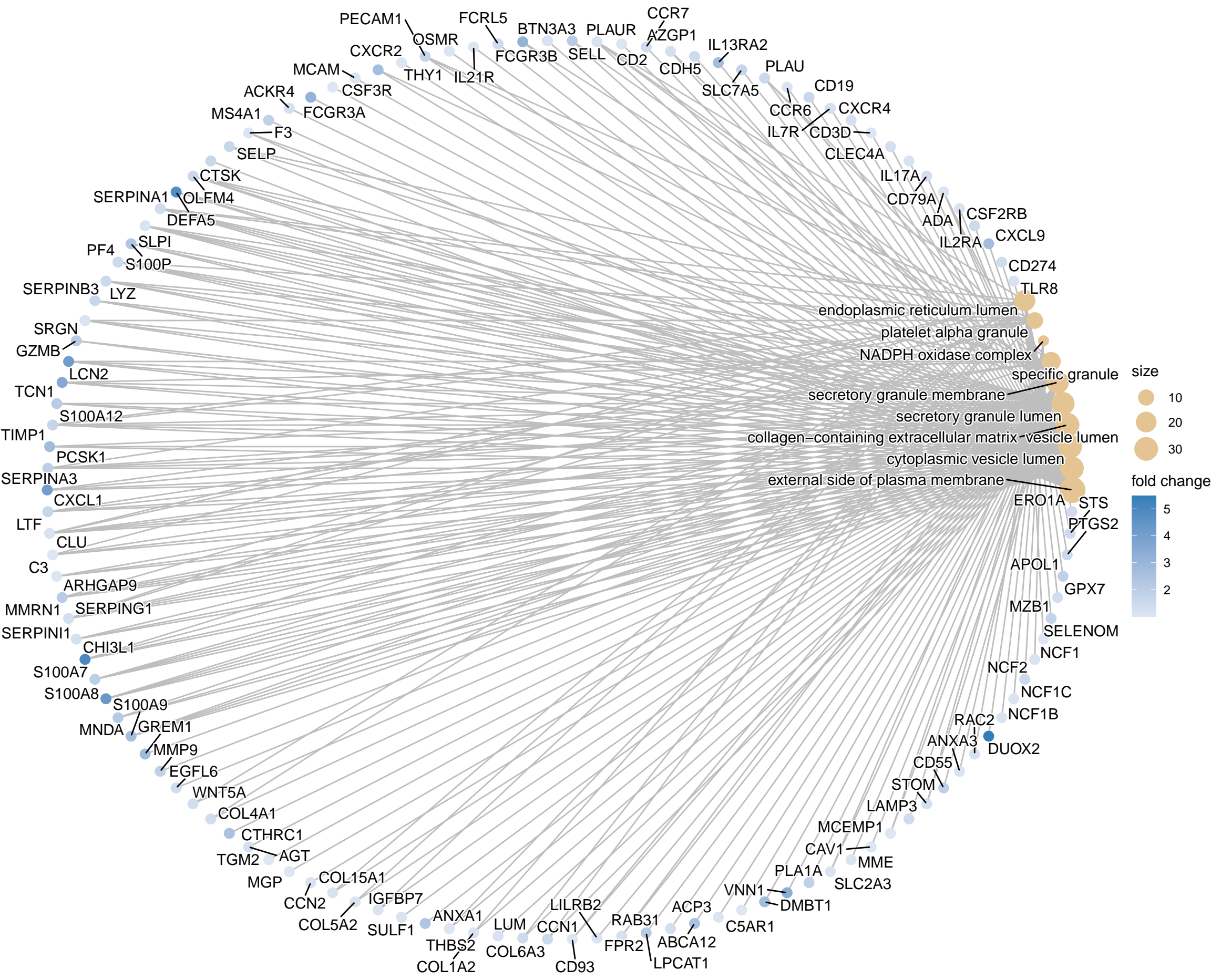
CC Cnetplot
