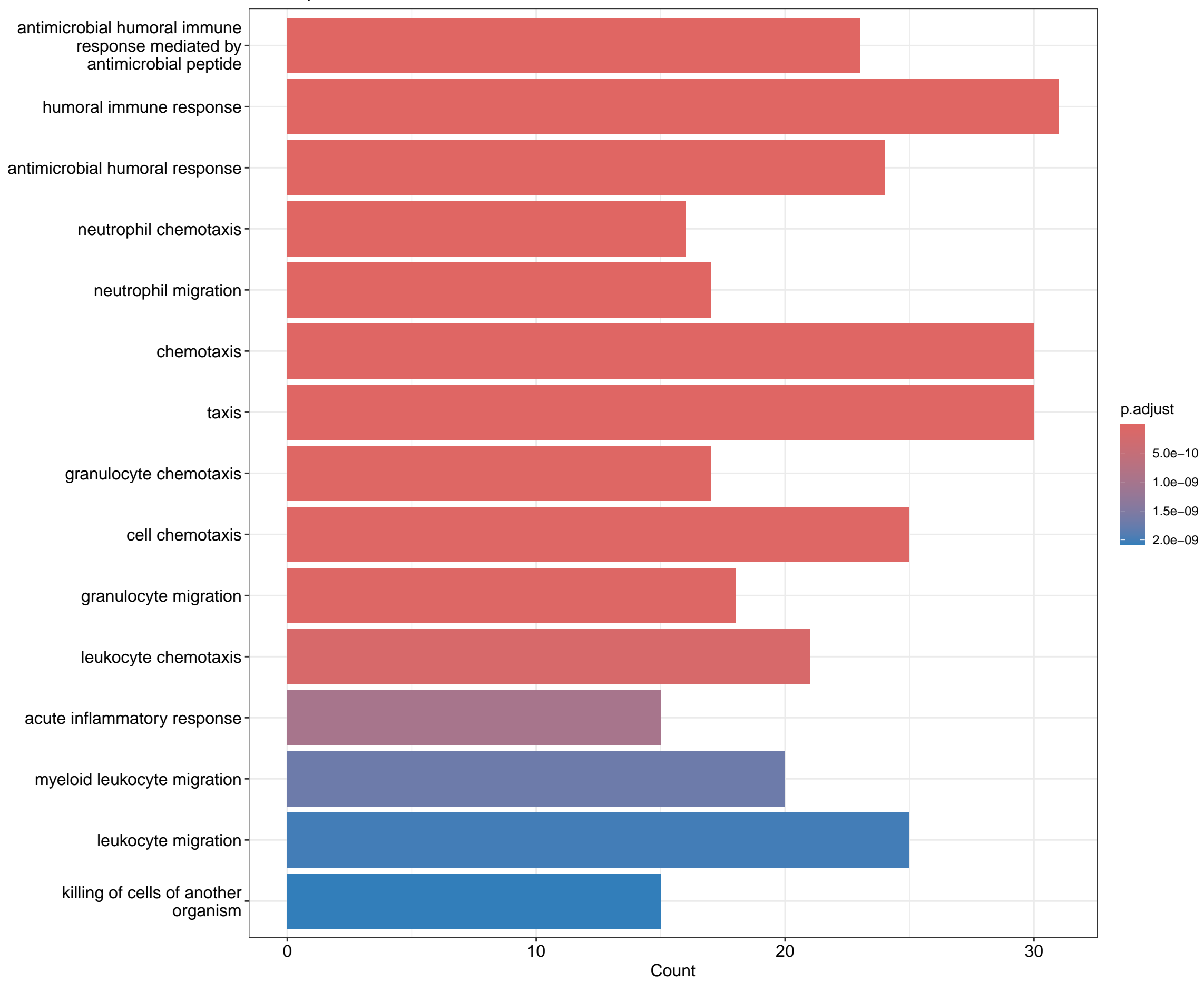
BP Barplot
