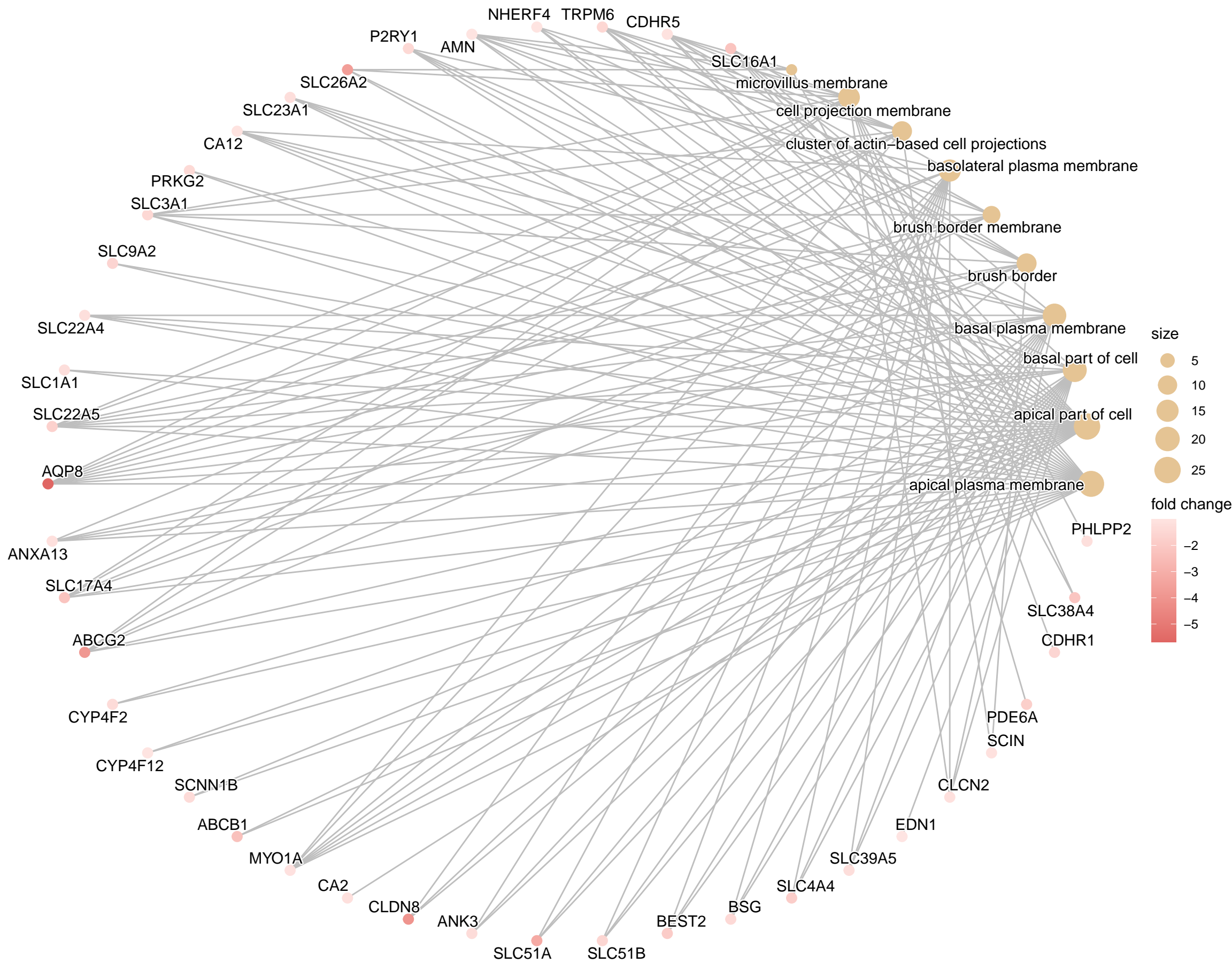
CC Cnetplot
