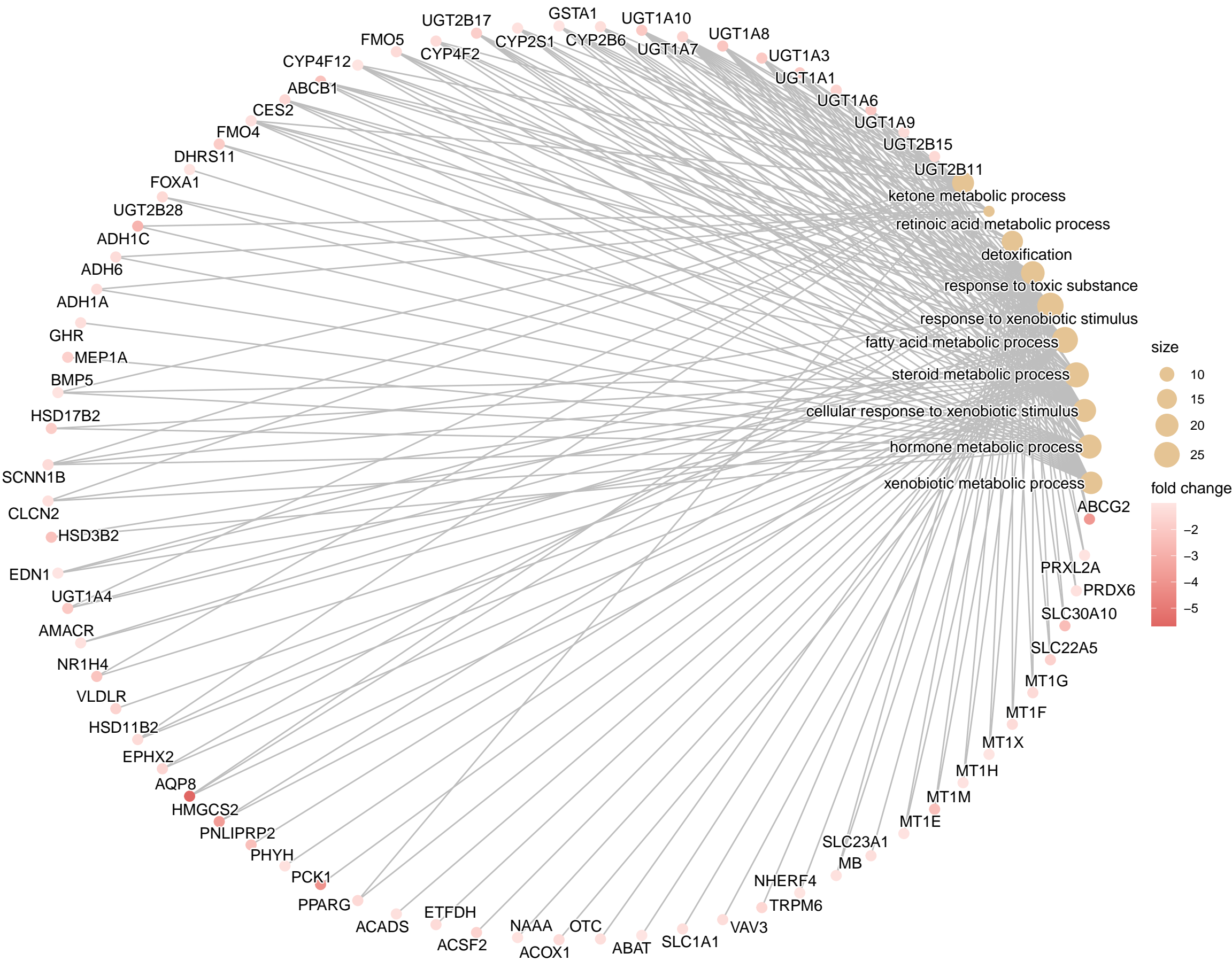
BP Cnetplot
