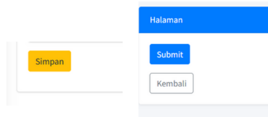
Gambar 9. Menyimpan Jawaban
