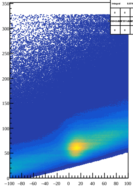
Prompt
