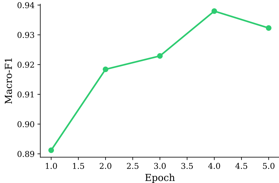
Validation Macro-F1
