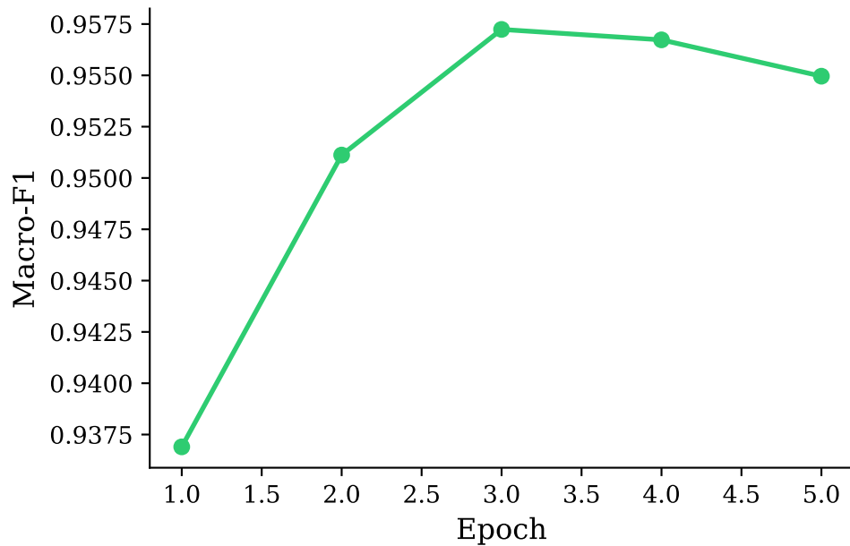
Validation Macro-F1
