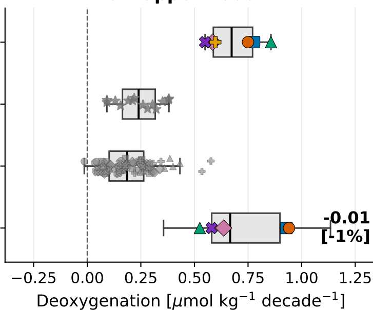
d. Upper 2000m
