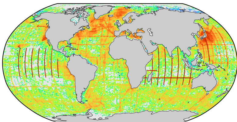
f) 8x sampling
