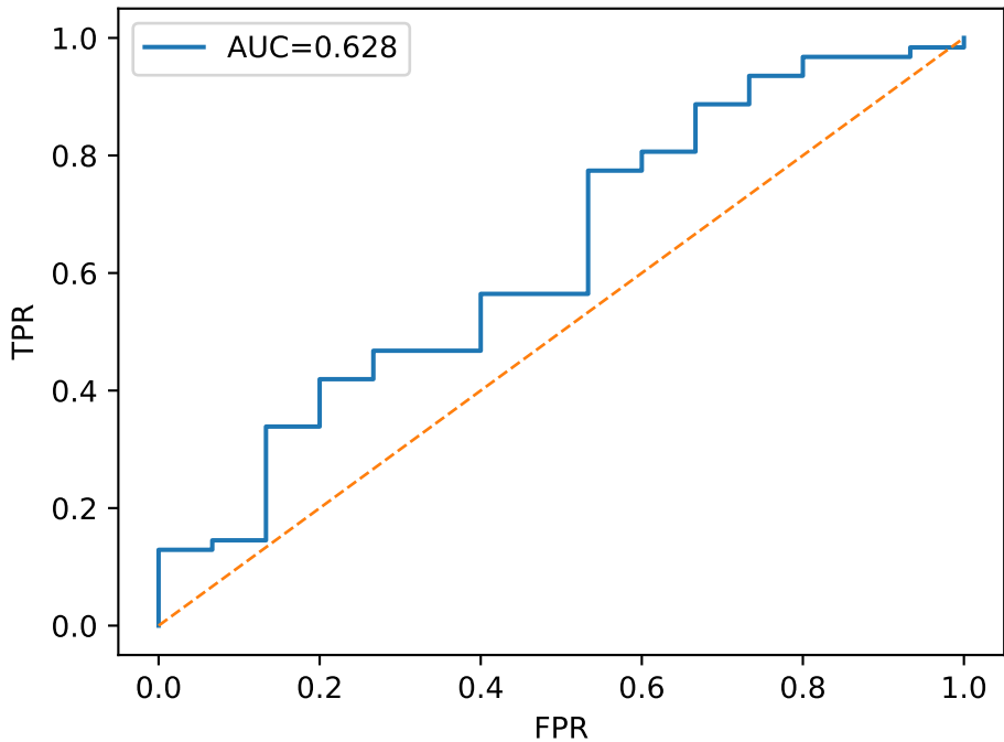
ROC (val)
