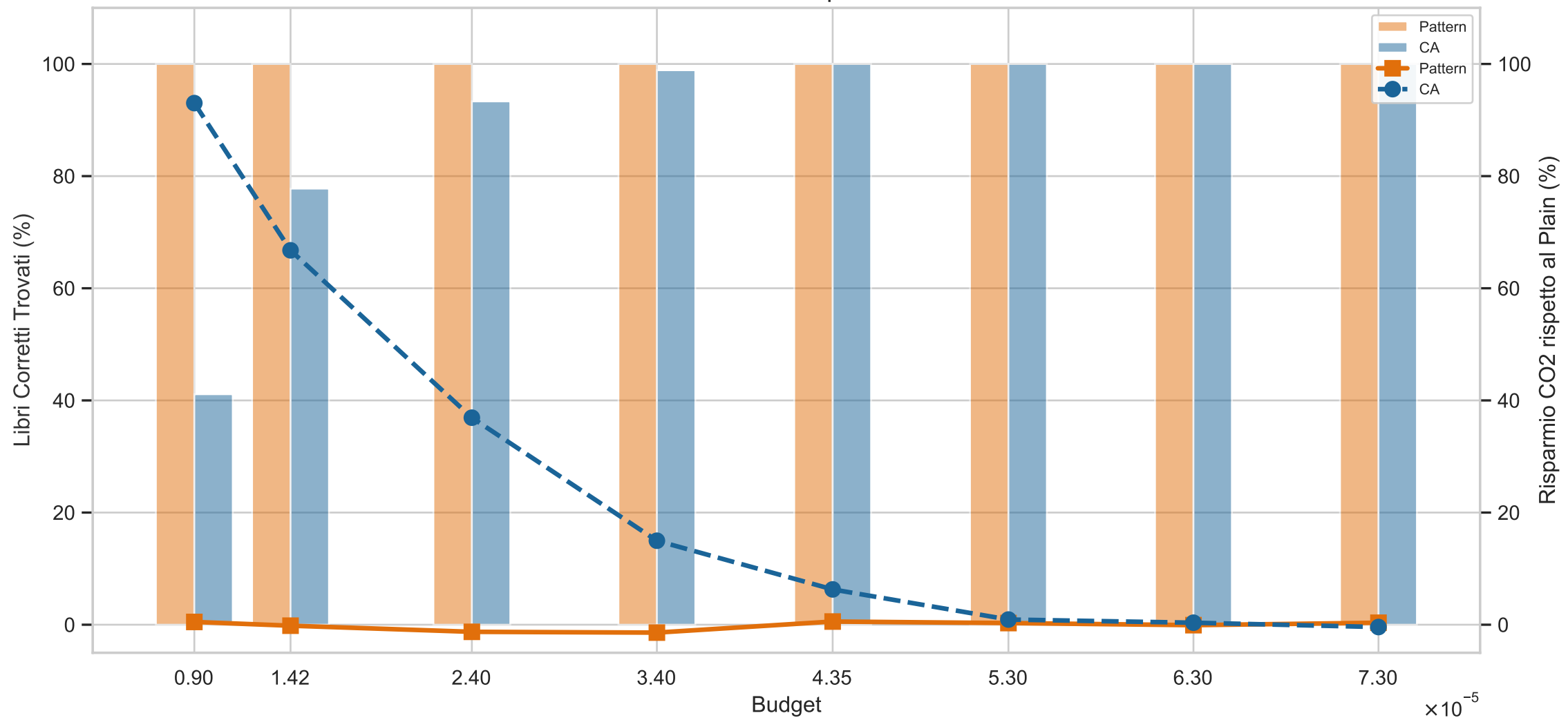
Accuratezza vs Risparmio CO2
