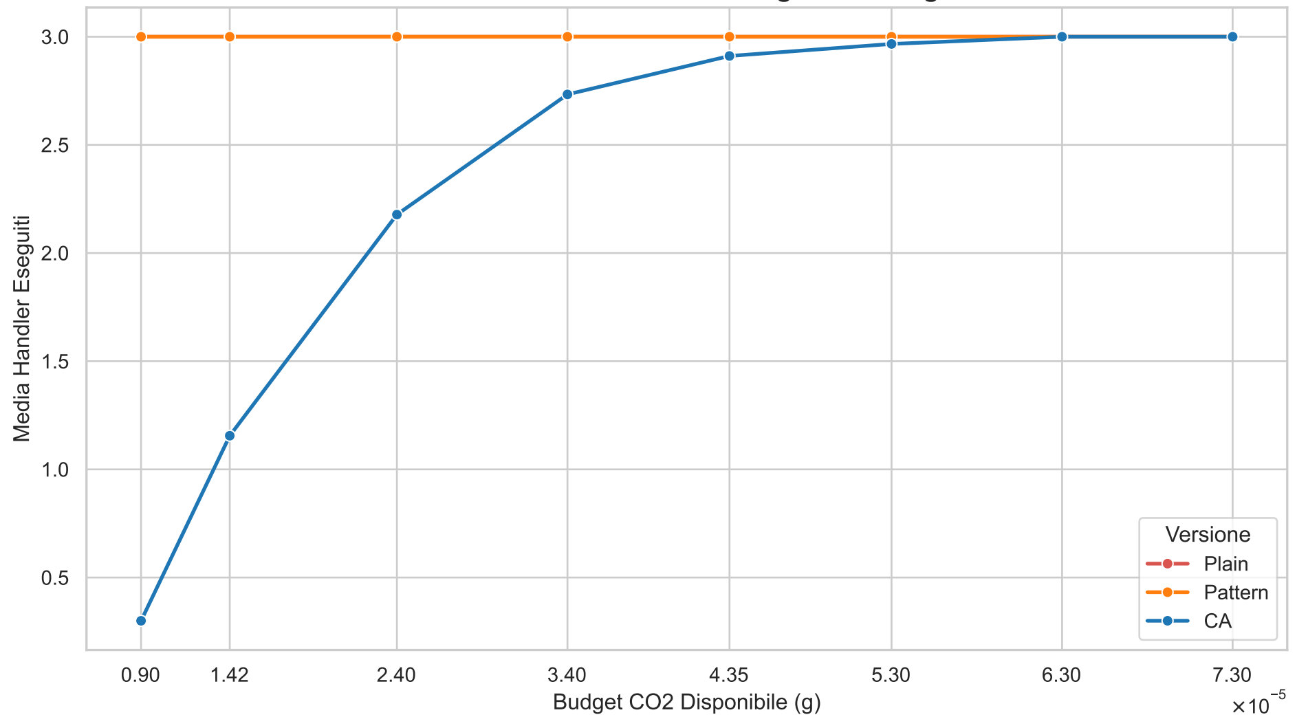
Numero Medio di Handler Eseguiti vs Budget
