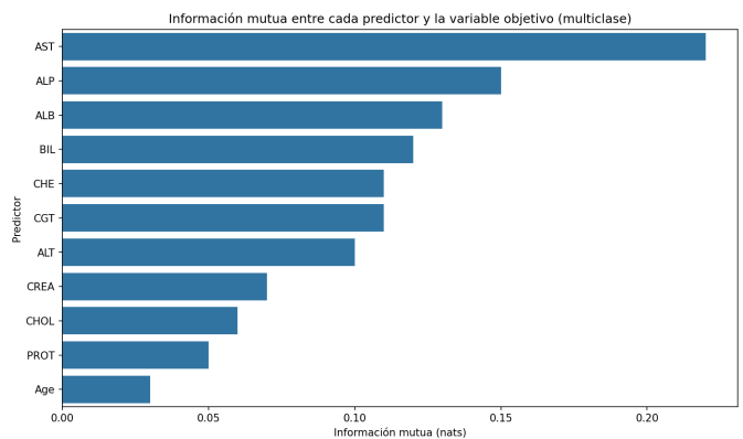
Figura 7. Información mutua entre las características y la variable respuesta (formulación multiclase).
