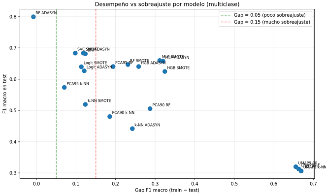
Figura 1. Desempeño vs. sobreajuste por modelo (multiclase). Eje x : gap F_1 macro train–test (mayor = más sobreajuste). Eje y : F_1 macro en test. La región ideal es la esquina superior izquierda (alto F_1 , gap pequeño).
