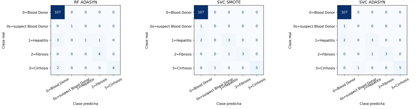
Figura 3. Matrices de confusión de los tres mejores modelos en test por F_1 macro (multiclase). Eje x : clase predicha. Eje y : clase real.
