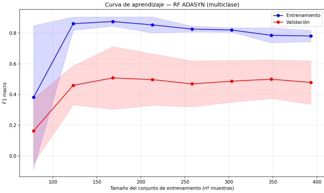
Figura 2. Curva de aprendizaje del mejor modelo (RF ADASYN, multiclase). Eje x : número de muestras de entrenamiento. Eje y : F_1 macro. Bandas: \pm 1\sigma sobre 5 folds.
