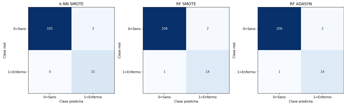
Figura 4. Matrices de confusión de los tres mejores modelos en test por F_1 macro (binario). Eje x : clase predicha. Eje y : clase real.
