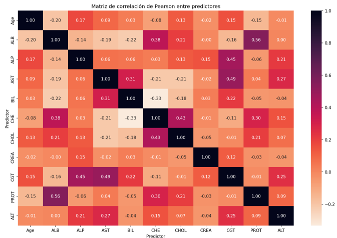
Figura 6. Matriz de correlación lineal de Pearson para el conjunto de características.
