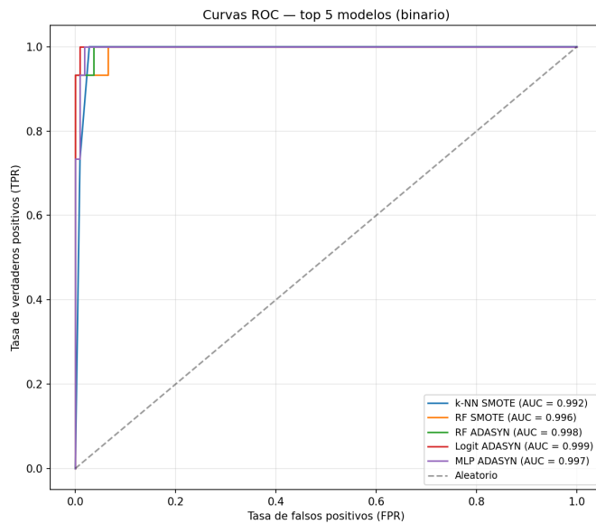
Figura 5. Curvas ROC superpuestas para los cinco mejores modelos (binario). Eje x : tasa de falsos positivos. Eje y : tasa de verdaderos positivos. AUC reportado en la leyenda.
