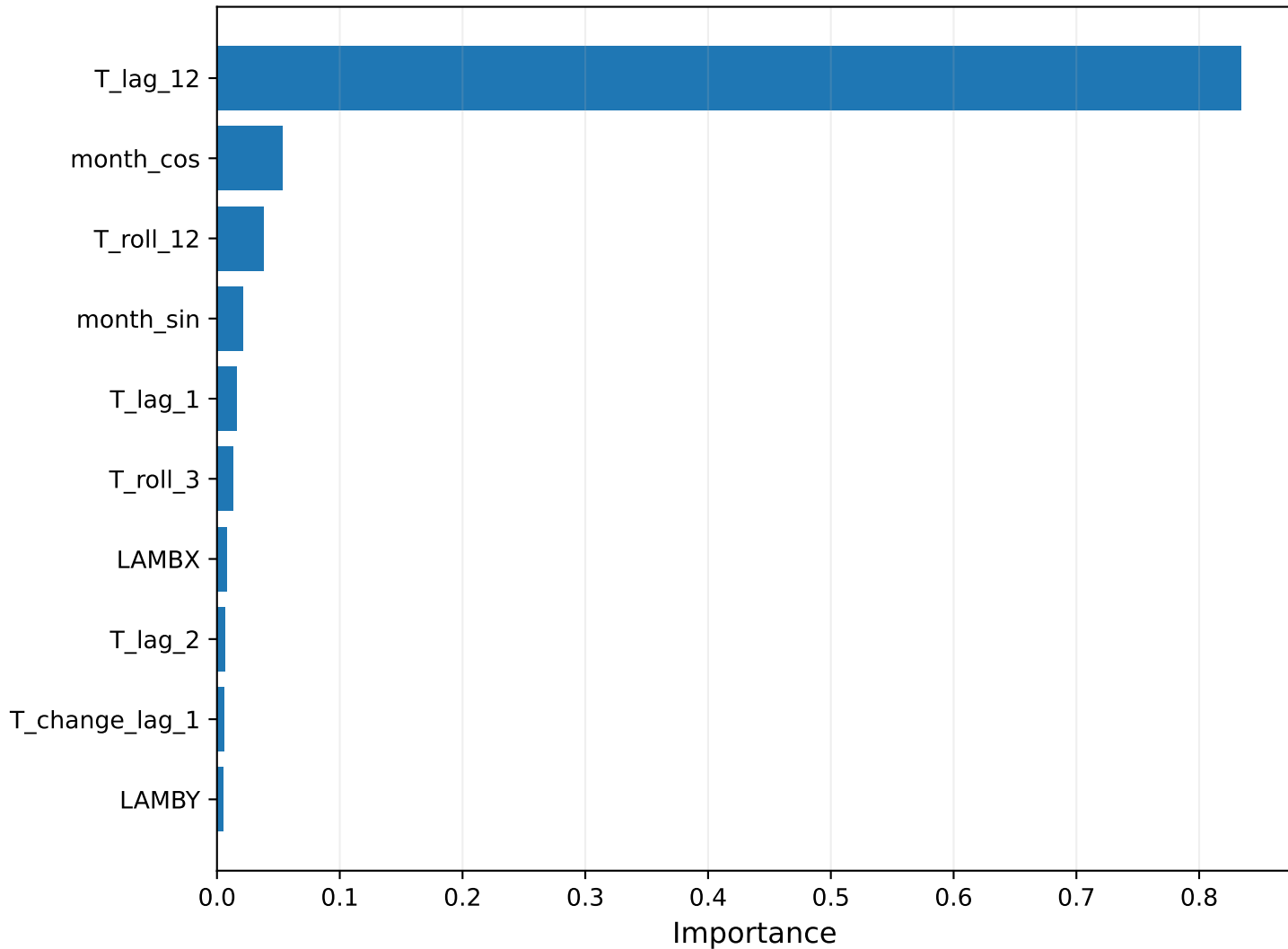
Importance des variables XGBoost
