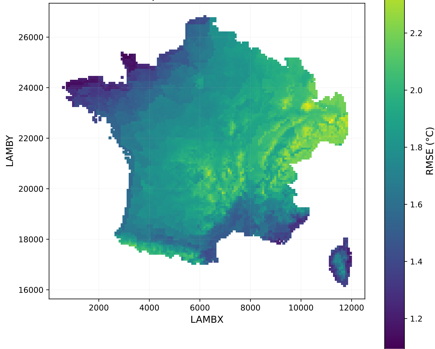
RMSE spatiale du modèle XGBoost
