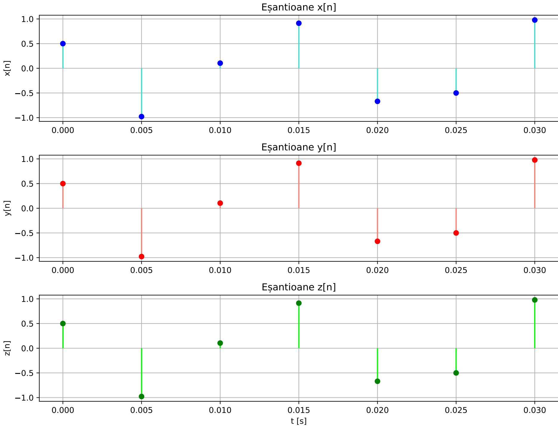
(c) Semnale Eșantionate la f_s = 200 Hz
