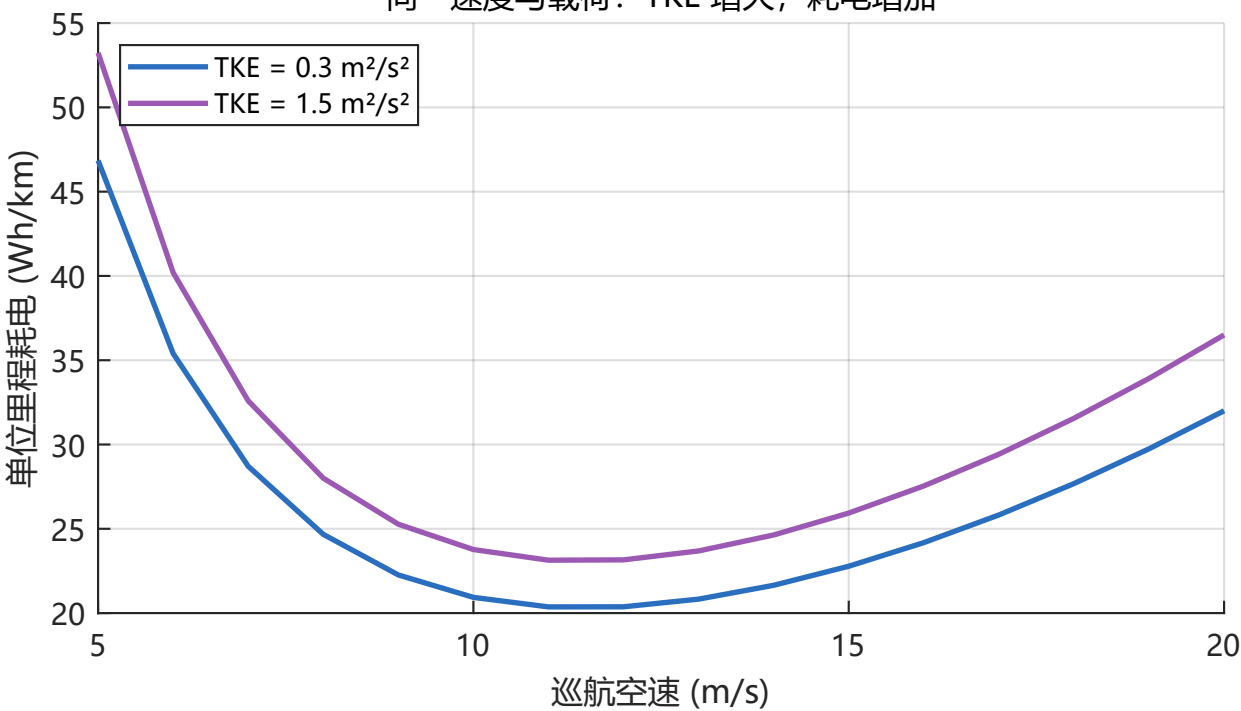
同一速度与载荷：TKE 增大，耗电增加
