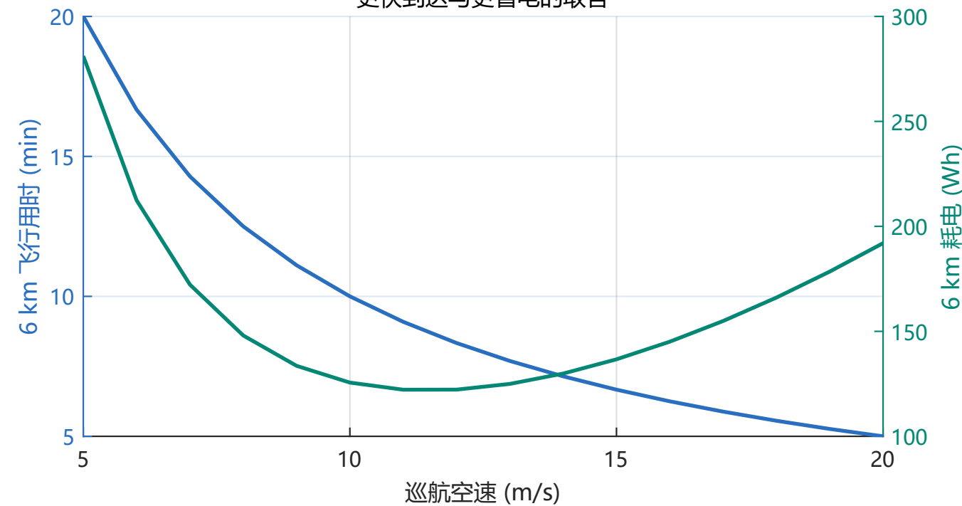
更快到达与更省电的取舍
