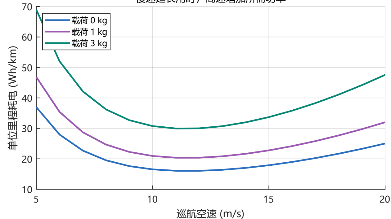
更快到达与更省电的取舍
