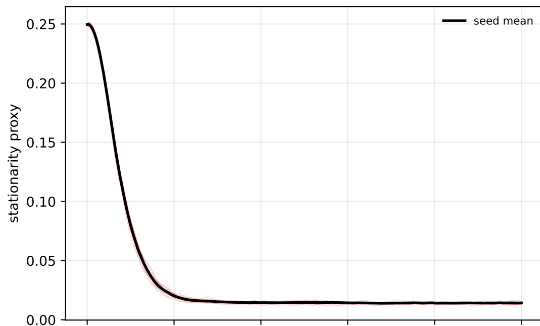
DGFM+
