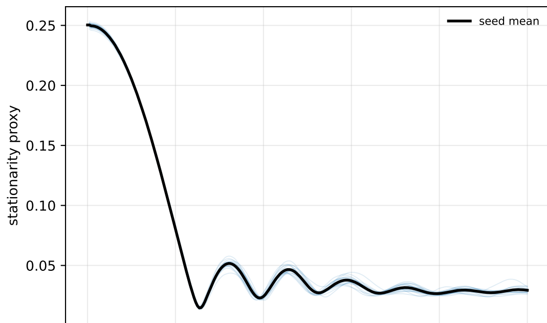
NOG-ZO
