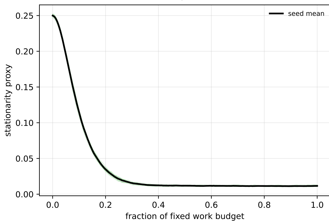
DGFM
