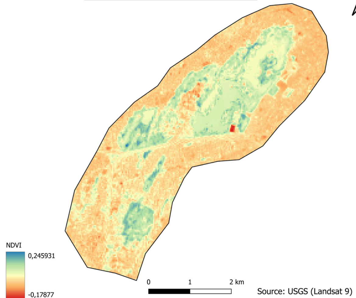
NDVI de 2024
