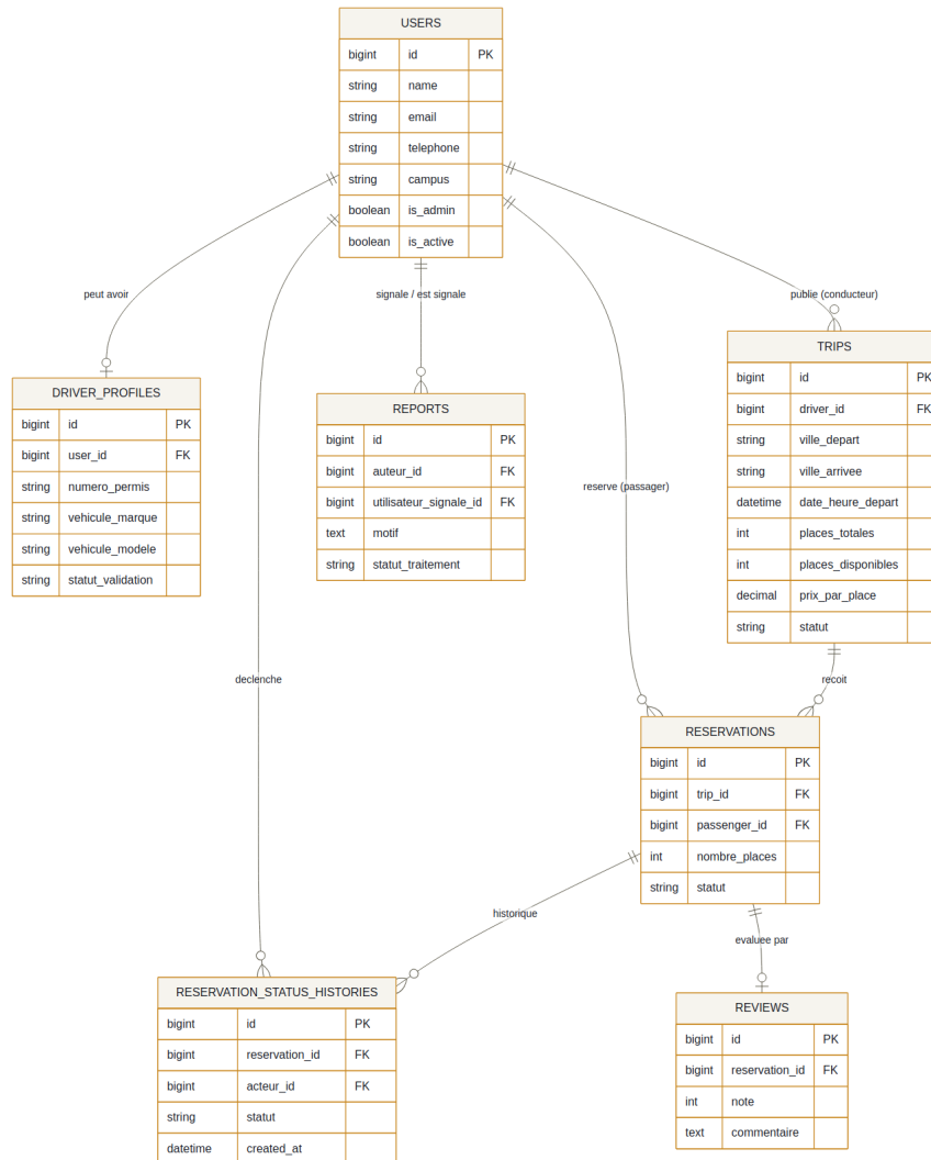
Figure 2 — Modèle relationnel simplifié
