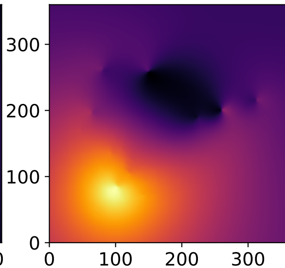
Abell 2744
