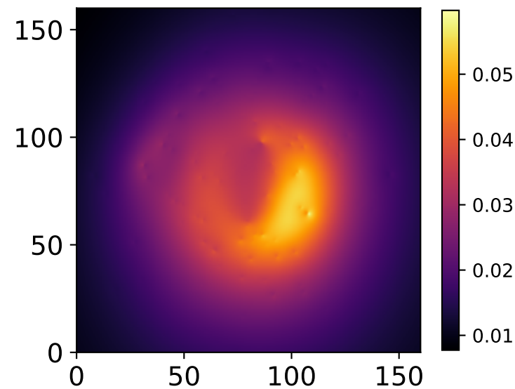
Abell 370
