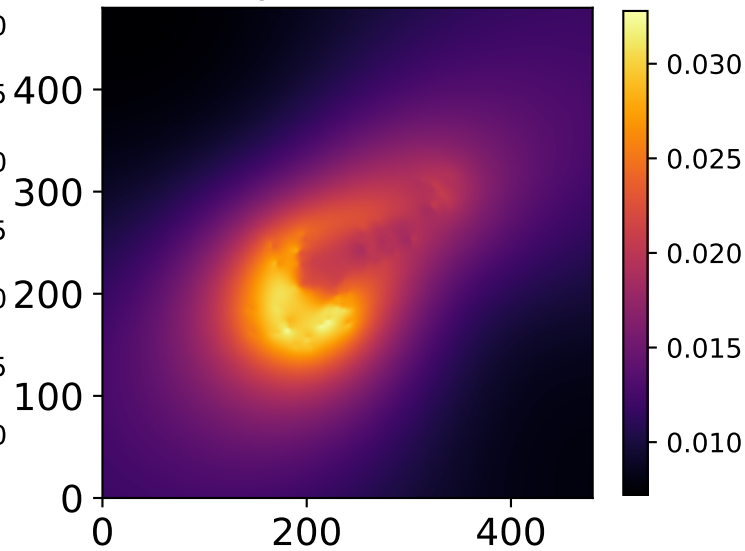
MACS J0717.5+3745
