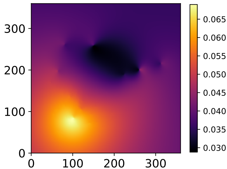
Abell 2744
