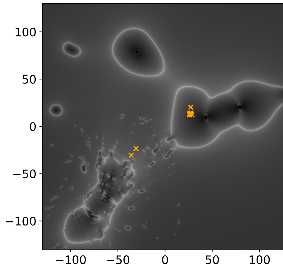
MACS J0717.5+3745
