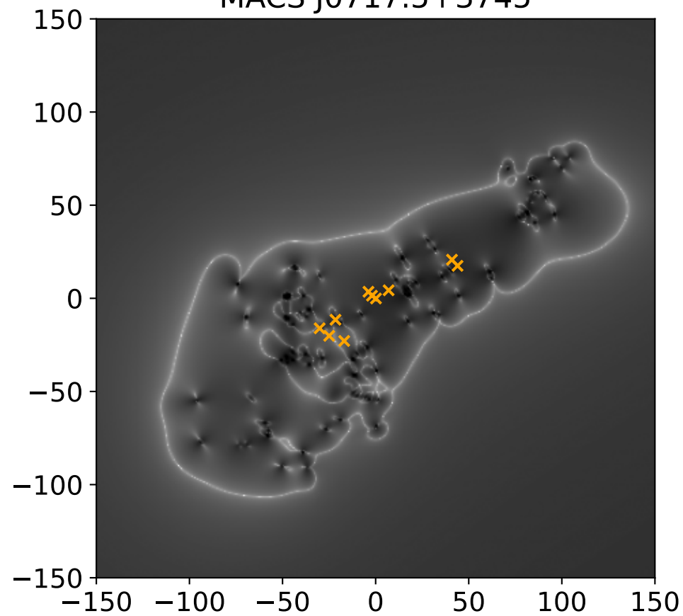
MACS J0717.5+3745
