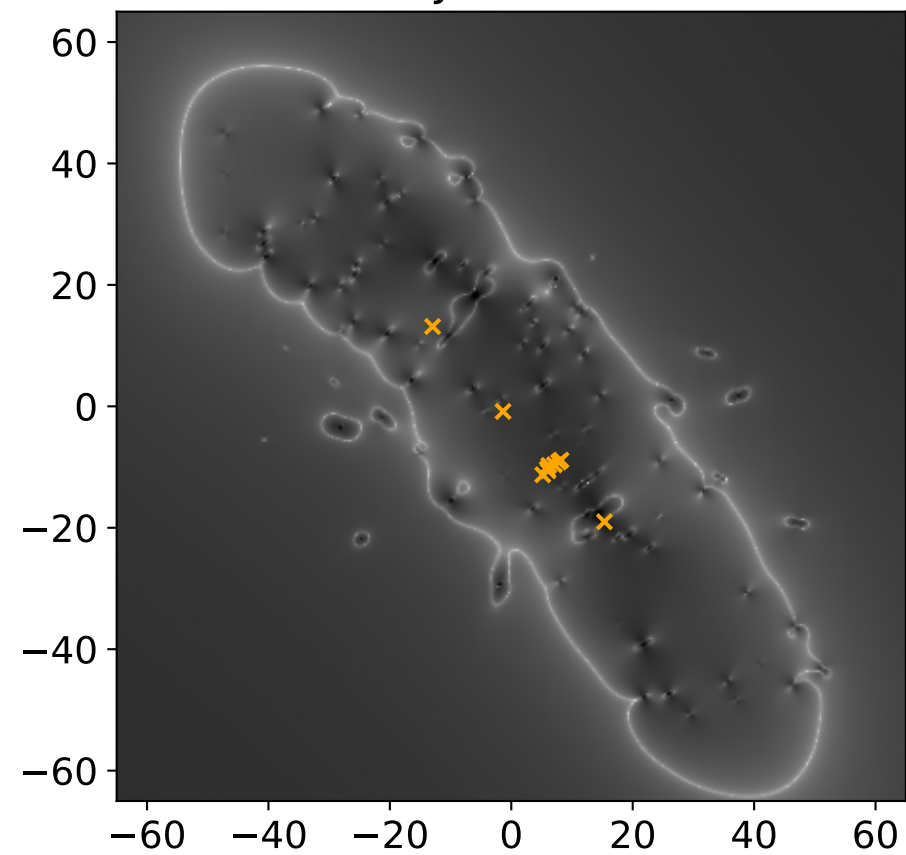
MACS J0416.1-2403
