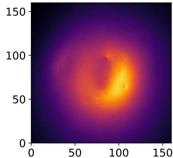
Abell 370
