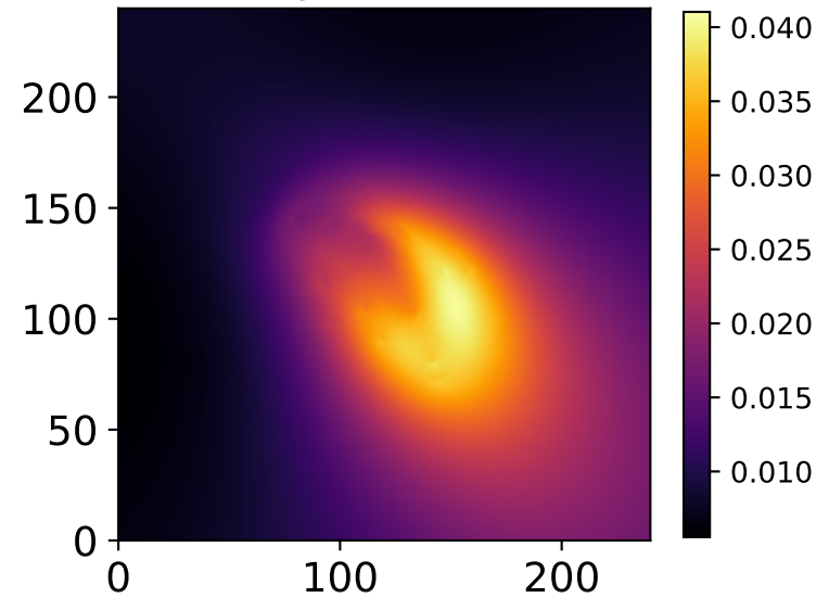
MACS J0416.1-2403
