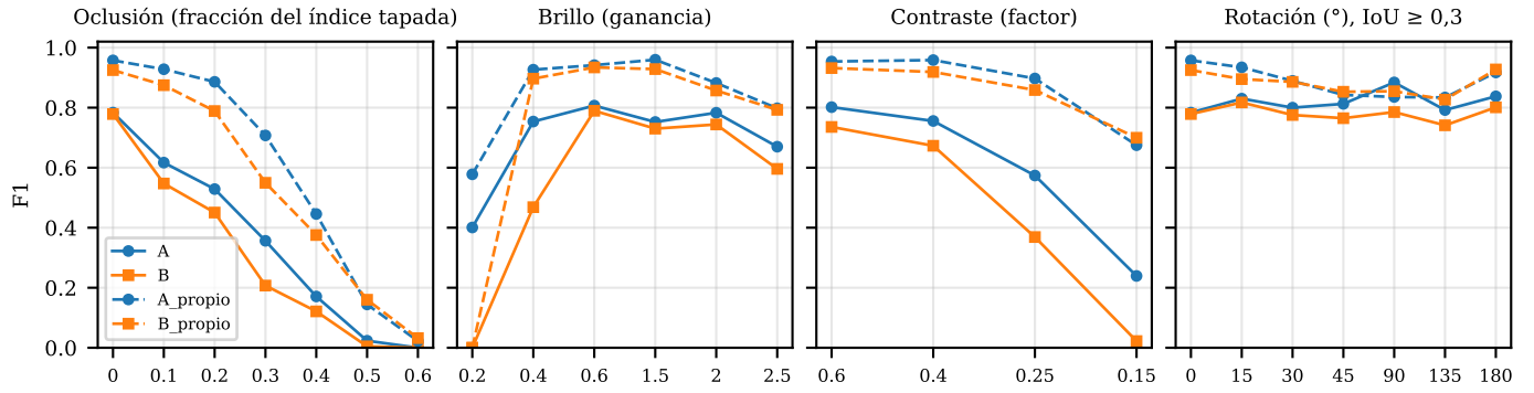
Figura 3. F1 en el test propio en función de la severidad de cada perturbación (trazo lleno: modelos base; trazo cortado: ajustados con fotos propias). Las rotaciones se miden con IoU \geq 0,3 (ver texto).
