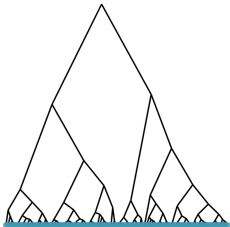
(d) Ward's linkage dendrogram
