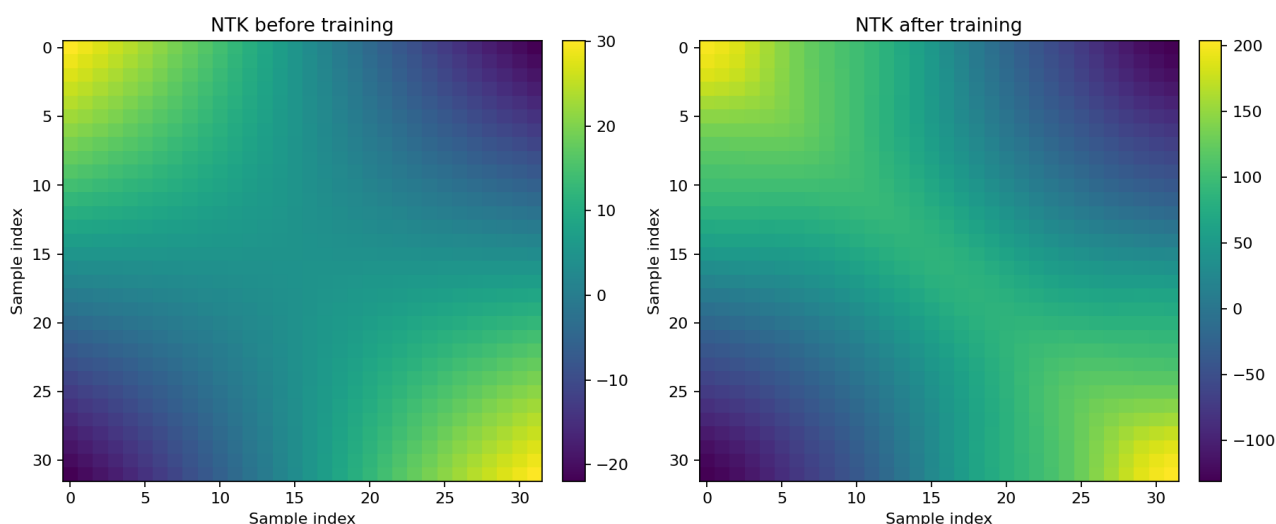
Рисунок 22 – Сравнение матриц NTK до и после обучения. До обучения ядро определяется в основном архитектурой и случайной инициализацией; после обучения структура NTK становится более контрастной, что отражает перераспределение чувствительности модели в соответствии с геометрией данных и целевой функцией.
