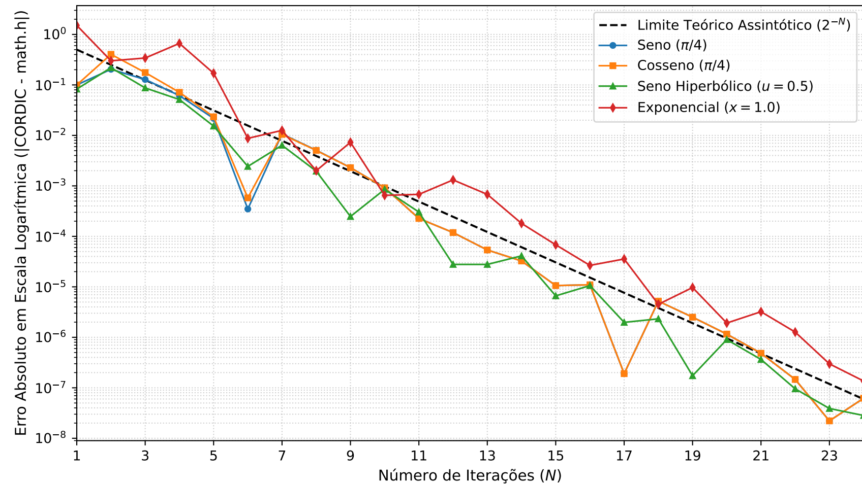
Convergência do Erro Absoluto do CORDIC vs. Limite Teórico
