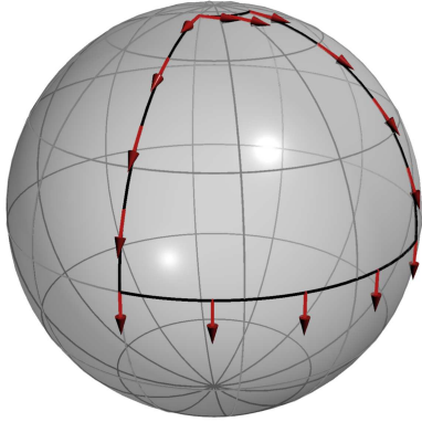
Figura 24: Transporte del vector \mathbf{u} = \partial_x = \partial_\theta a lo largo de la trayectoria marcada en negro. Durante los tres primeros tramos, las componentes del vector no se ven alteradas, de modo que tenemos siempre \mathbf{u} = \partial_\theta . En el último tramo cercano al polo norte sí se producen modificaciones en las componentes, de tal modo que al volver al punto de origen \mathbf{u} \approx \partial_y \propto \partial_p h i .
