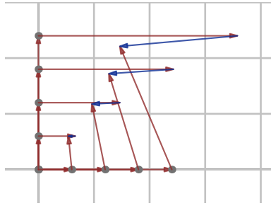
Figura 25: “Paralelogramos” abiertos dados por la conexión del ejemplo 22. Se muestran desplazamientos de norma 0.4, 0.3, 0.2 y 0.1 en ambas direcciones.
