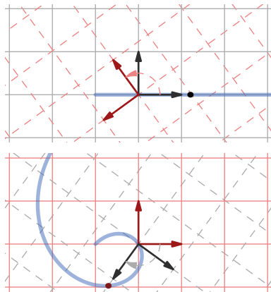
Figura 12: Trayectoria en ausencia de fuerzas externas. Las condiciones iniciales son x(0) = -1, y(0) = 0, v^x(0) = 1, v^y(0) = 0 . En la parte superior se toman las coordenadas grises, y se representa con línea punteada el sistema rotante en un instante dado por \omega t = 11/5 . En la parte inferior se representa la misma trayectoria vista desde el sistema rotante.
