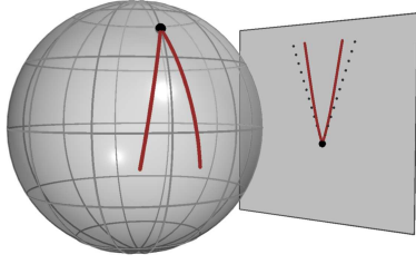
Figura 26: Cono (triángulo) geodésico en la esfera partiendo de un punto con coordenadas \theta = \pi/4 , \phi = \pi/3 . Las curvas rojas son geodésicas. En el plano de coordenadas las geodésicas son curvas que quedan dentro de las líneas rectas punteadas, tangentes a las geodésicas en el punto.
