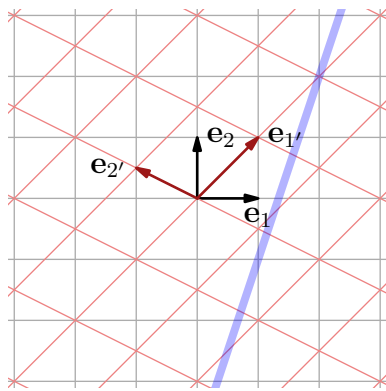
Figura 8: Igual que la fig. 4. Las líneas coordenadas de x^i (gris) y x^{i'} (rojo claro), acompañadas de los vectores de las bases asociadas a las coordenadas: \mathfrak{B} = \{e_i\}_{i=1}^2 y \mathfrak{B}' = \{e_{i'}\}_{i=1}^2 . Se añade una trayectoria rectilínea.
