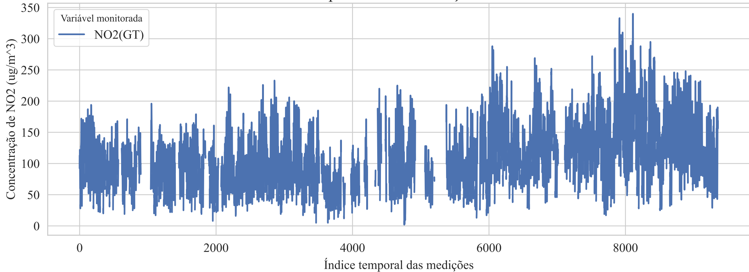
Série temporal da concentração de NO2
